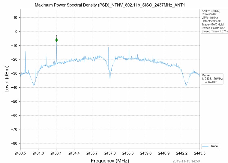
802.11b_2437MHz_SISO_ANT1
