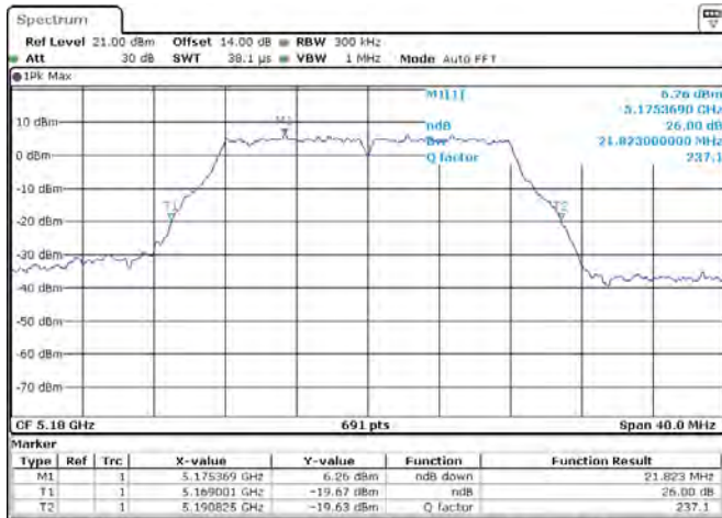
ANT 1(11A)
