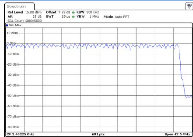
\pi/4 -DQPSK 2.4415 GHz ~ 2.4835 GHz
