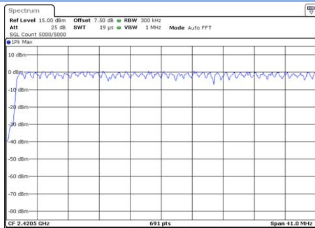
\pi/4 -DQPSK 2.4 GHz ~ 2.4415 GHz
