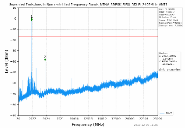
30MHz-25GHz CH00
