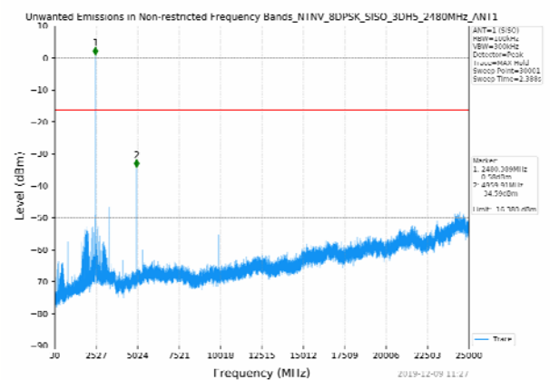
30MHz-25GHz CH78
