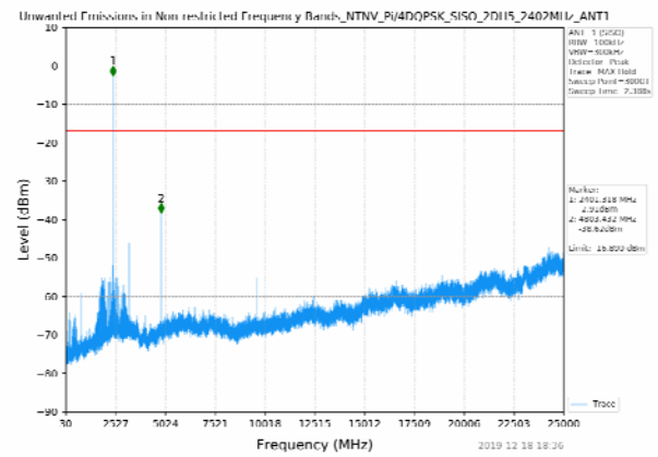
30MHz-25GHz CH00
