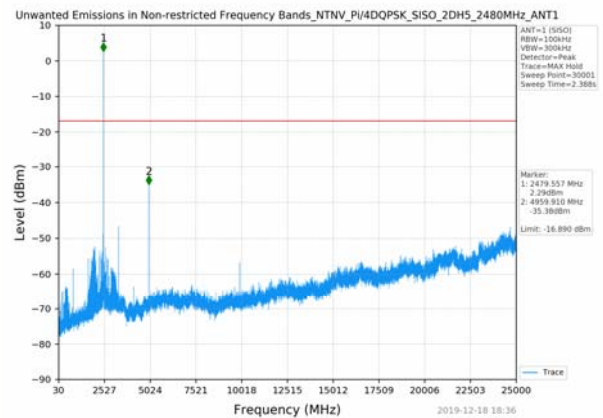
30MHz-25GHz CH78
