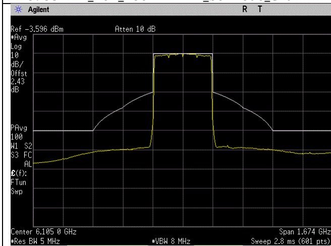
6105MHz_31_320MHz BW_be-mode_Chain 0
