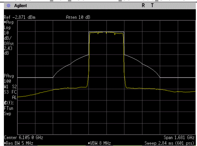
6105MHz_31_320MHz BW_be-mode_Chain 1
