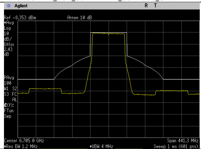
6705MHz_151_80MHz BW_be-mode_Chain 3
