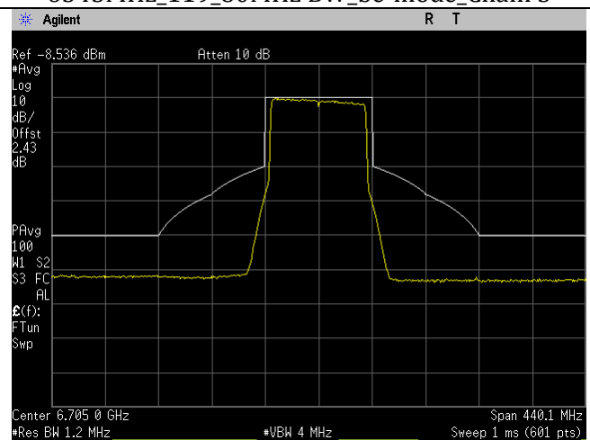
6705MHz_151_80MHz BW_be-mode_Chain 1
