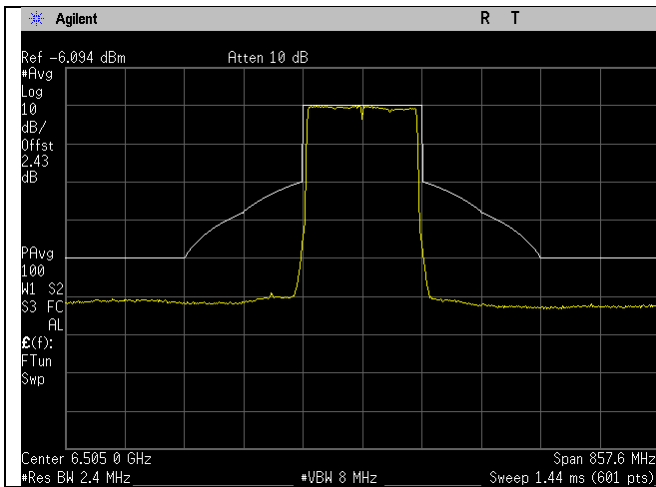
6505MHz_111_160MHz BW_be-mode_Chain 0
