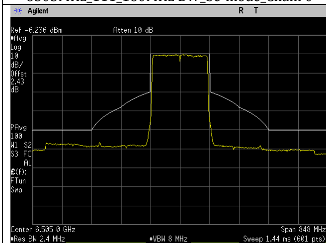
6505MHz_111_160MHz BW_be-mode_Chain 2
