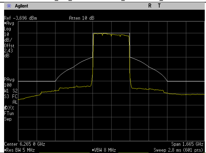
6265MHz_63_320MHz BW_be-mode_Chain 3
