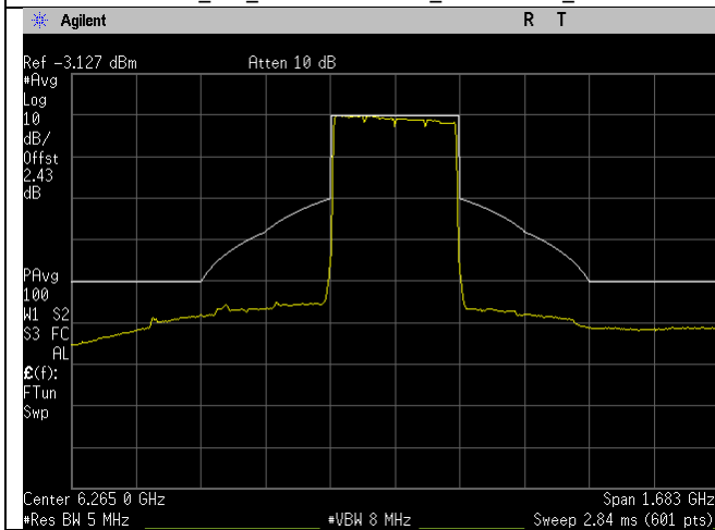
6265MHz_63_320MHz BW_be-mode_Chain 2
