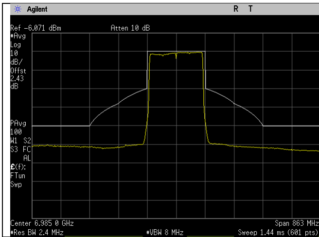
6985MHz_207_160MHz BW_be-mode_Chain 0
