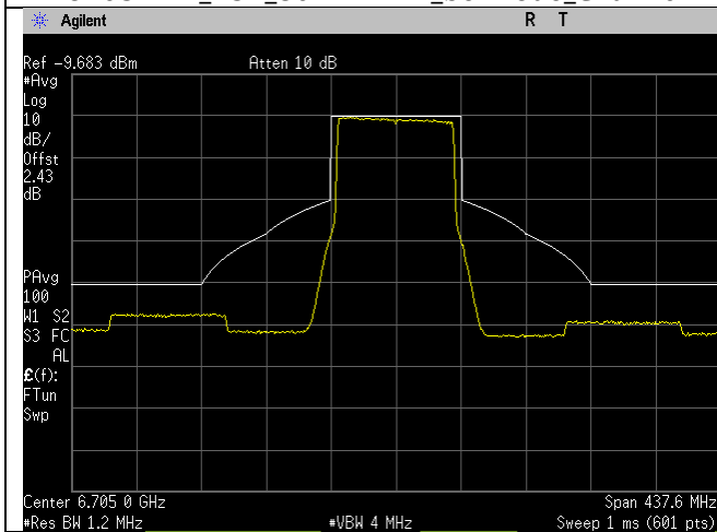
6705MHz_151_80MHz BW_be-mode_Chain 2
