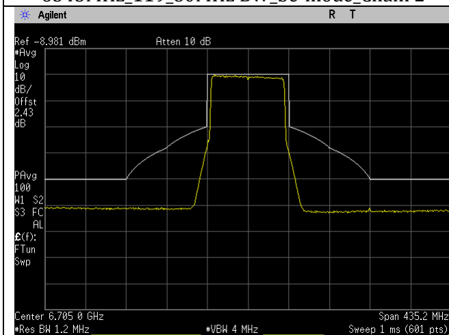
6705MHz_151_80MHz BW_be-mode_Chain 0
