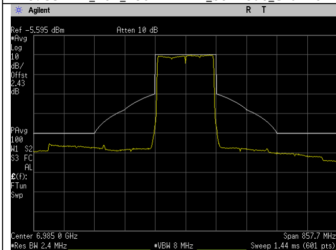
6985MHz_207_160MHz BW_be-mode_Chain 2
