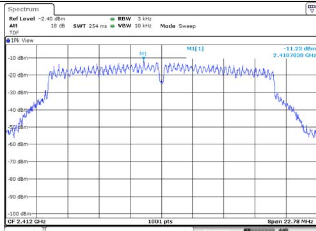
802.11g / 2 412 MHz
