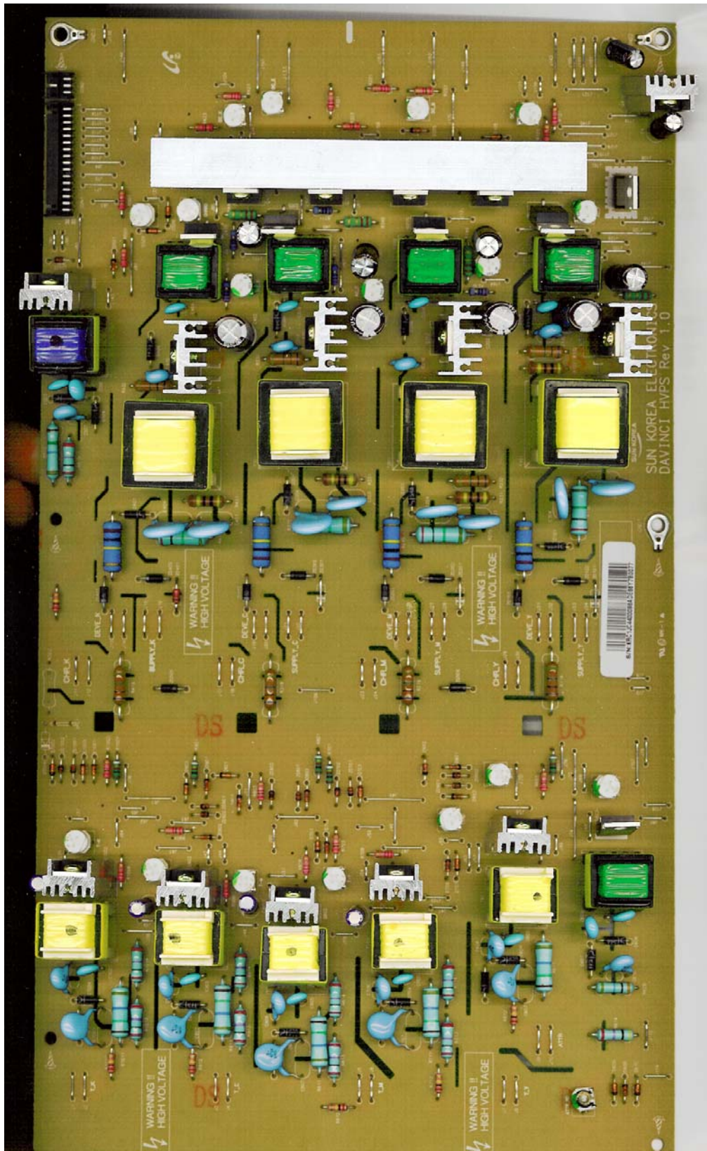
Fig. 05 HVPS PBA
