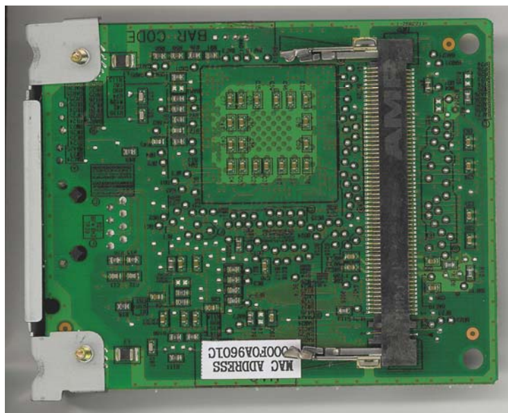
Fig. 14 NPC Solder
