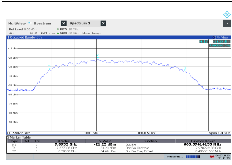
SP3_Preamble 9
