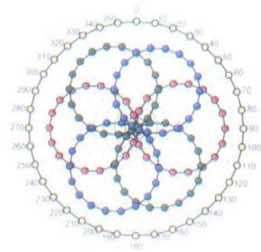
f = 600 MHz, TEM ifi110EXX
