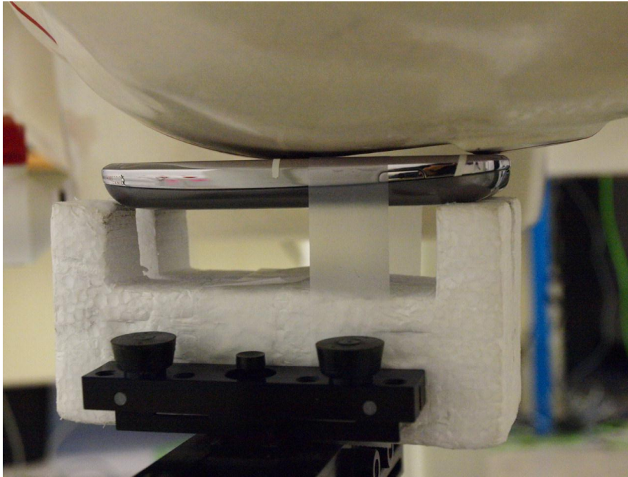
Left Tilt (15°)
