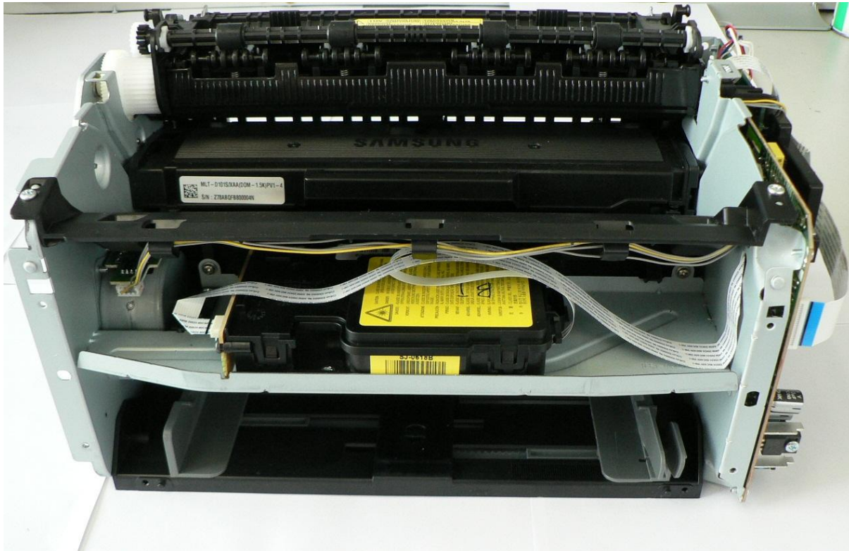
ML-2164W Printer_Front
