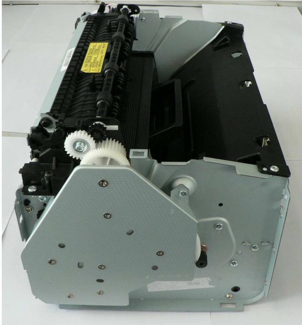
ML-2164W SIDE_RIGHT
