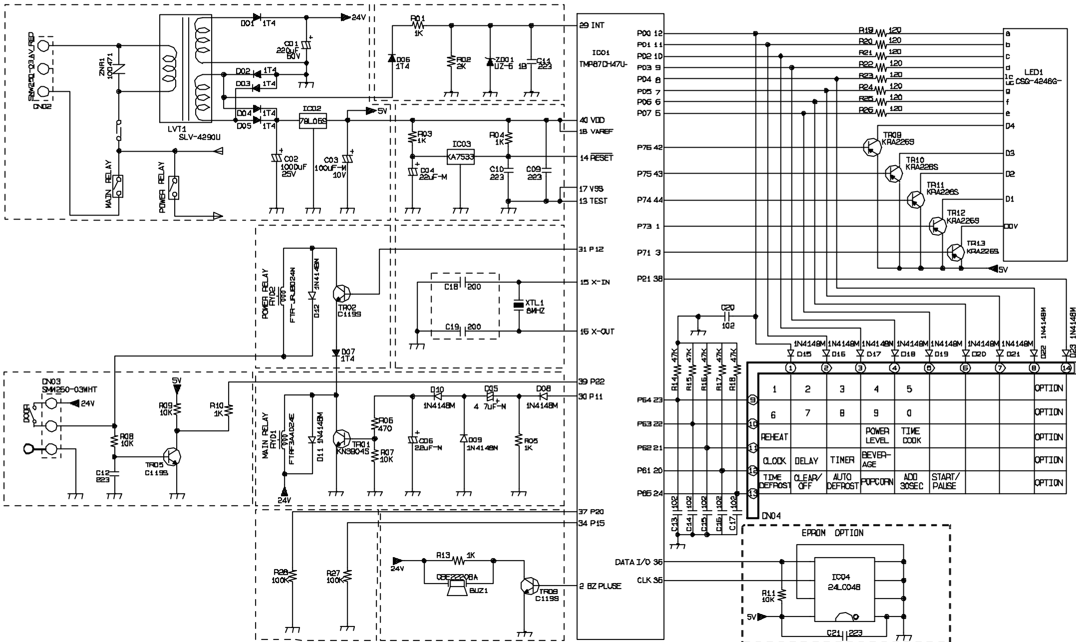
N2LED1 JES636WD SCHEMATIC
