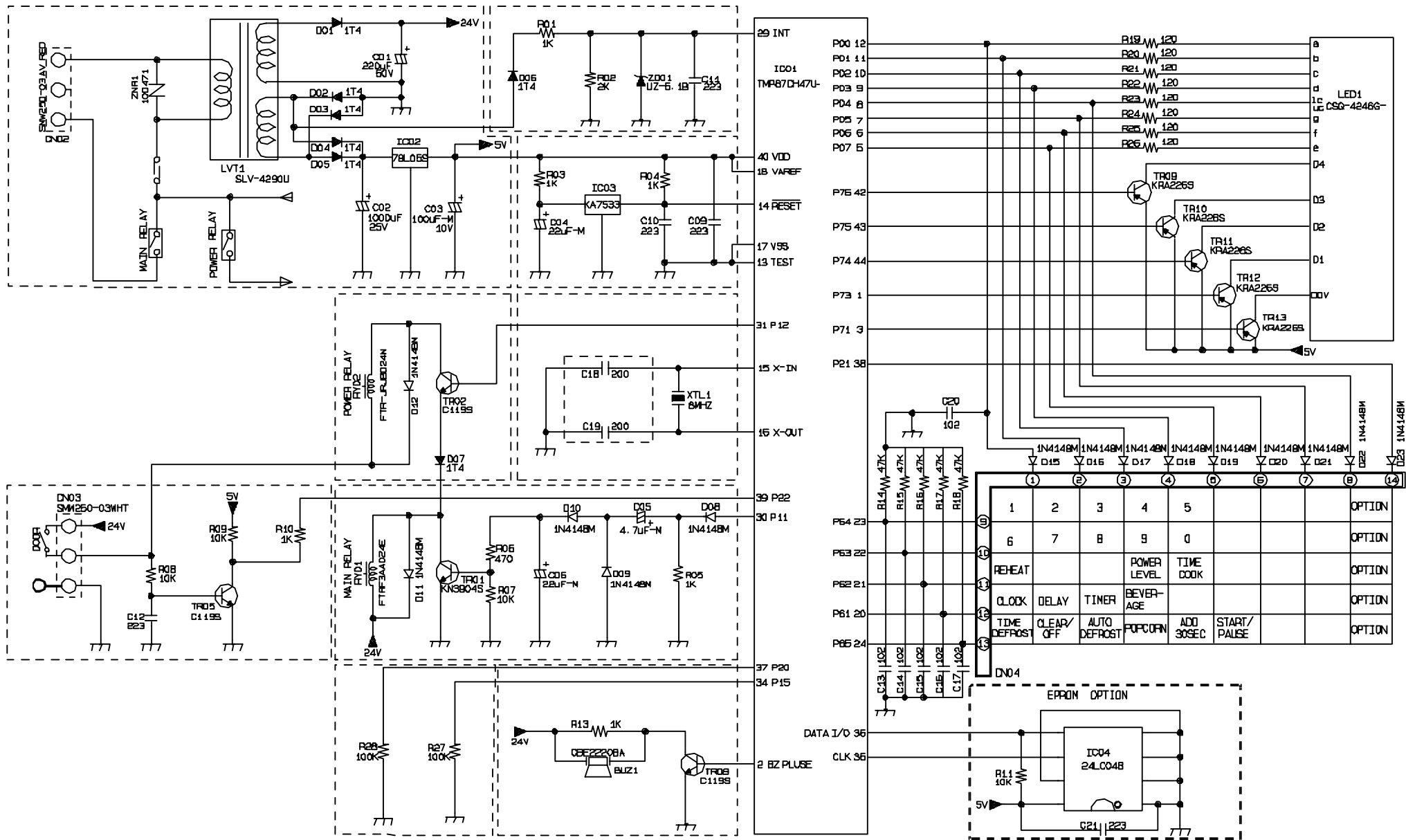
N2LED1 JES636WD SCHEMATIC
