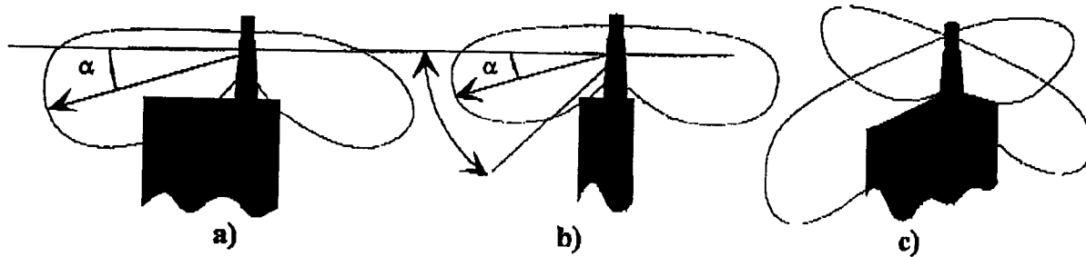
Figure 3.5.1 Radiation patterns, a) E1-plane (YZ-plane) b) E2-plane (XZ-plane) c) 3-D view
