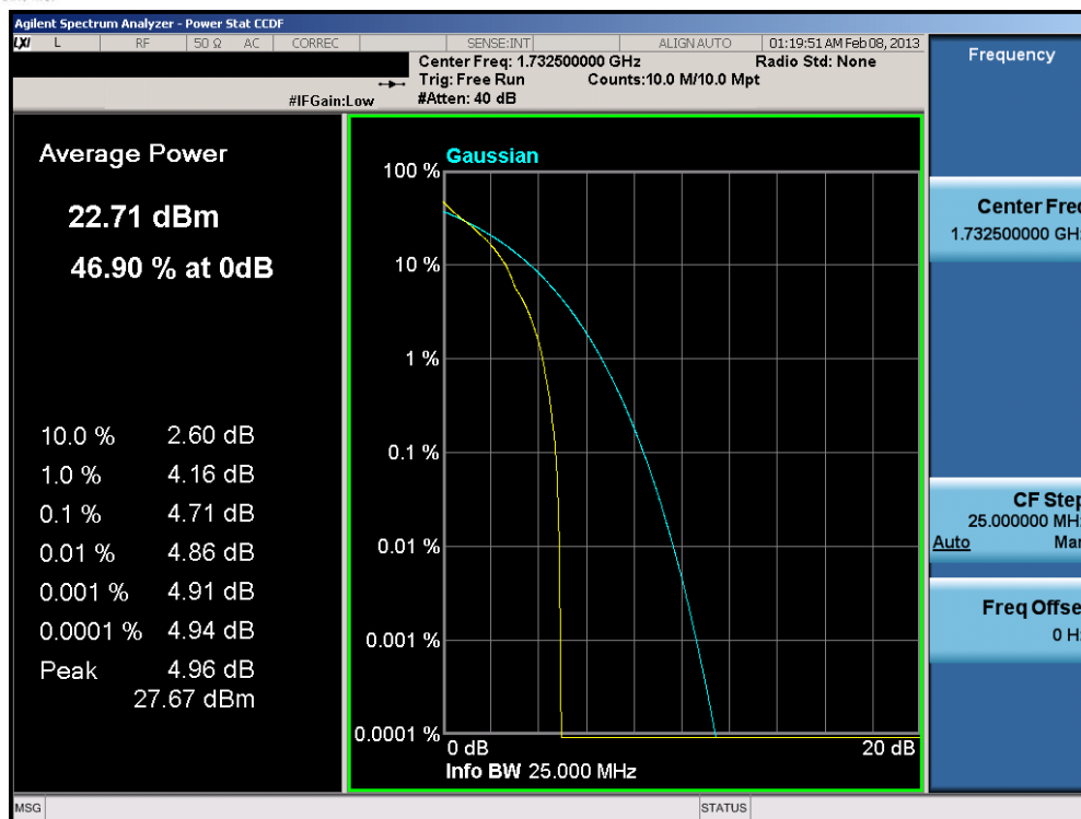
Plot 8-55. PAR Plot (20.0MHz QPSK – RB Size 100)
