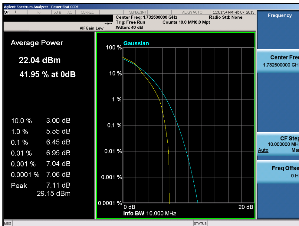
Plot 8-28. PAR Plot (10.0MHz 16-QAM – RB Size 50)
