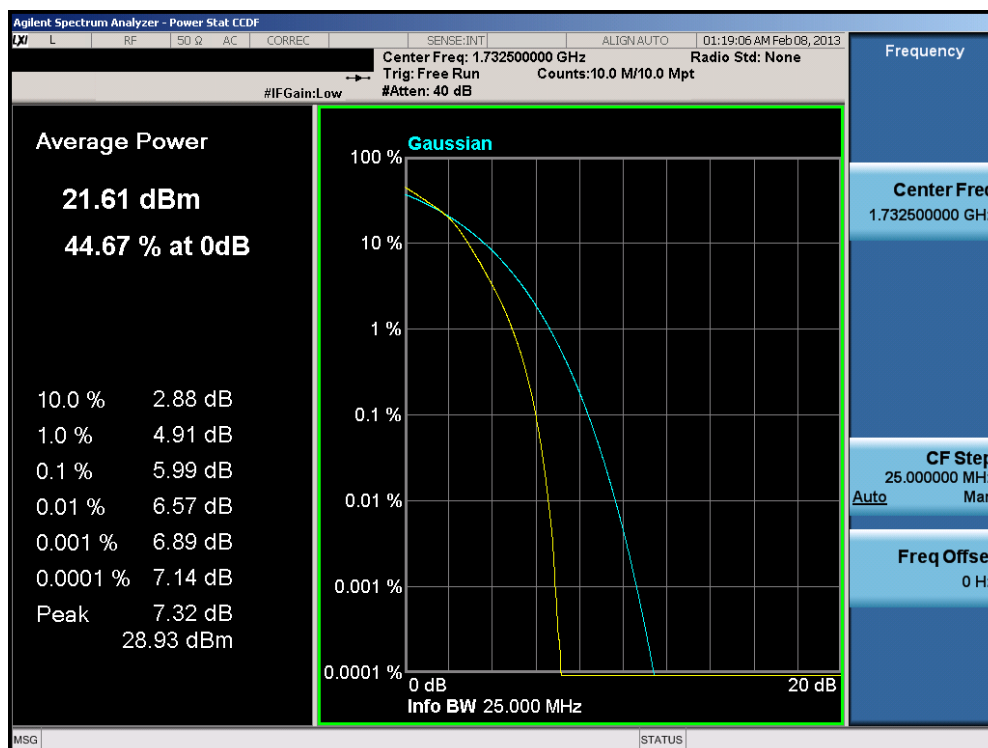
Plot 8-56. PAR Plot (20.0MHz 16-QAM – RB Size 100)
