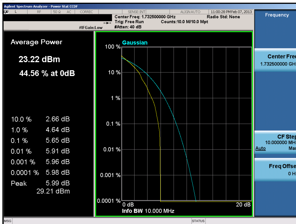
Plot 8-27. PAR Plot (10.0MHz QPSK – RB Size 50)
