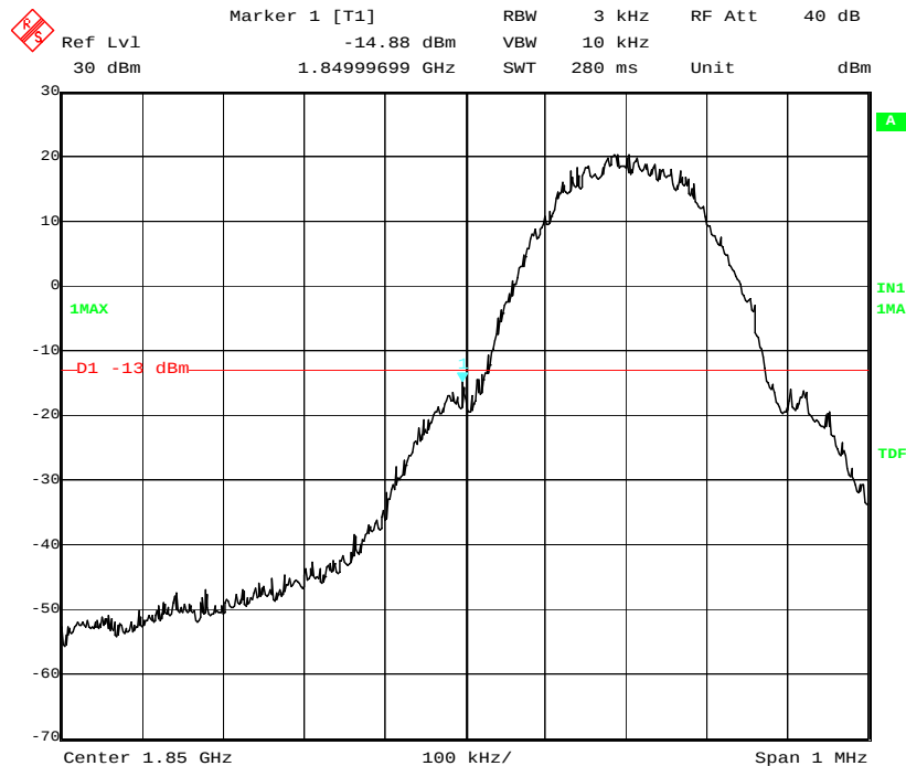
Low channel band edge
