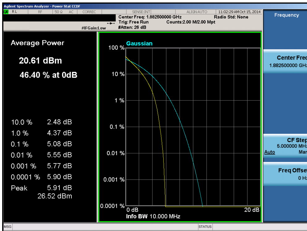
Plot 6-108. PAR Plot (Band 25 – 10.0MHz QPSK – RB Size 50)
