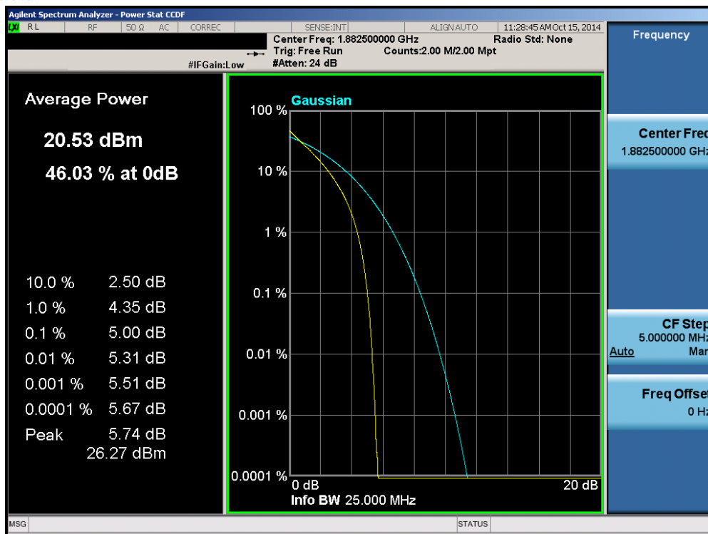
Plot 6-110. PAR Plot (Band 25 – 15.0MHz QPSK – RB Size 75)
