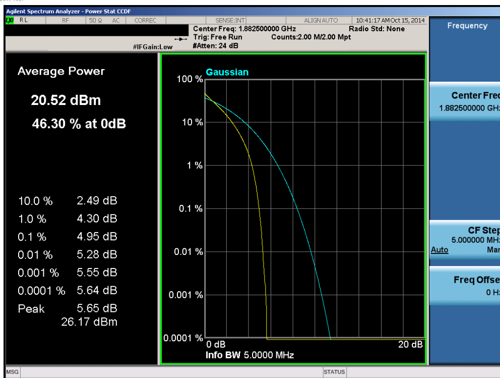
Plot 6-106. PAR Plot (Band 25 – 5.0MHz QPSK – RB Size 25)
