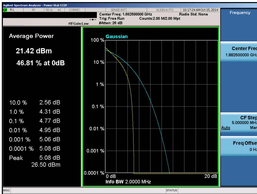
Plot 6-102. PAR Plot (Band 25 – 1.4MHz QPSK – RB Size 6)
