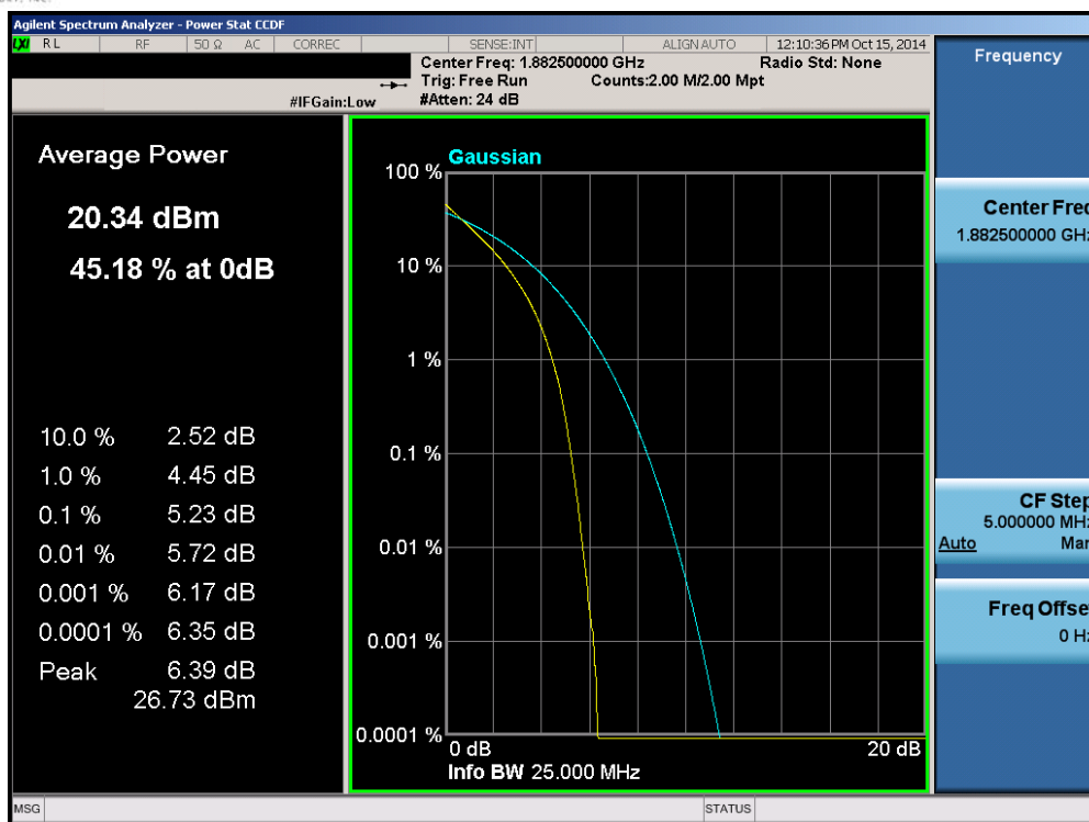
Plot 6-112. PAR Plot (Band 25 – 20.0MHz QPSK – RB Size 100)
