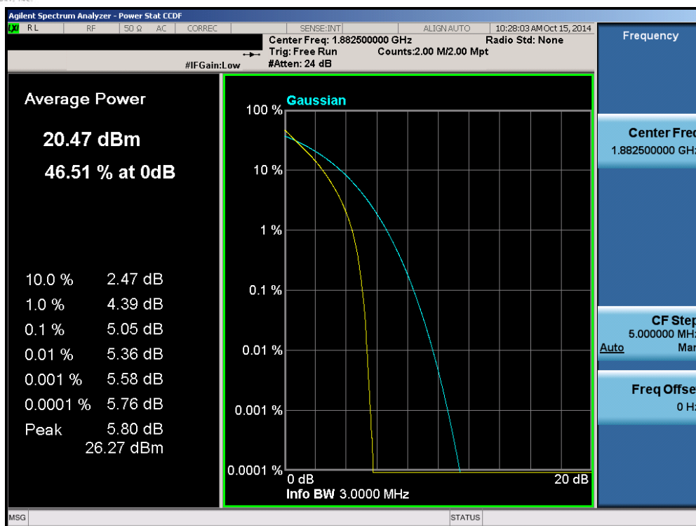
Plot 6-104. PAR Plot (Band 25 – 3.0MHz QPSK – RB Size 15)
