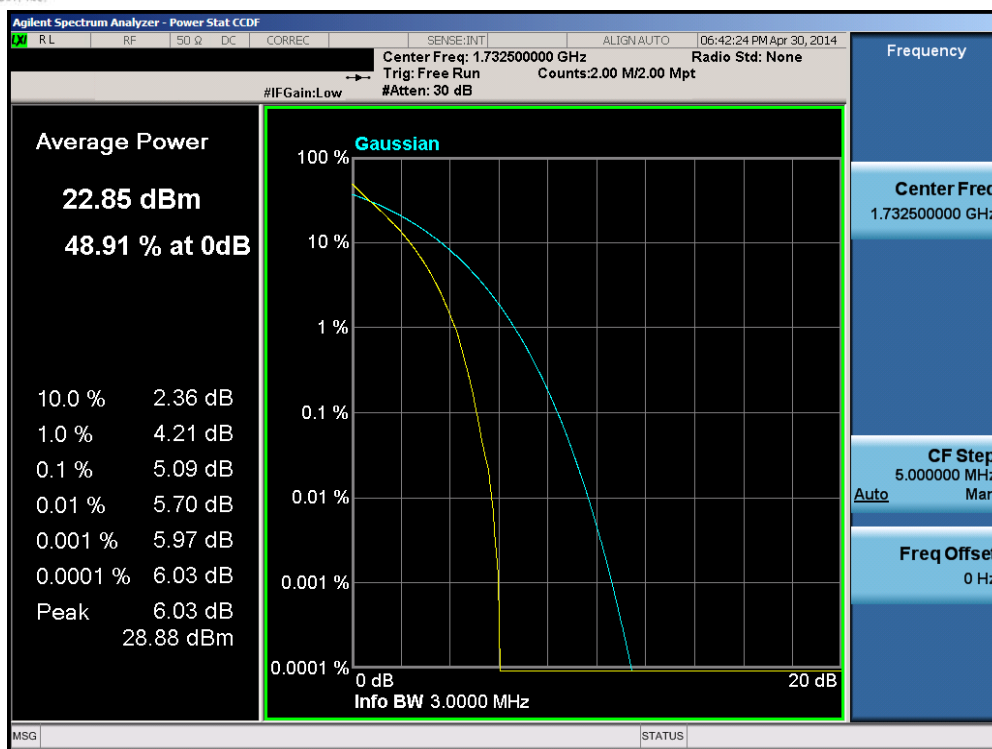
Plot 6-147. PAR Plot (Band 4 – 3.0MHz QPSK – RB Size 15)
