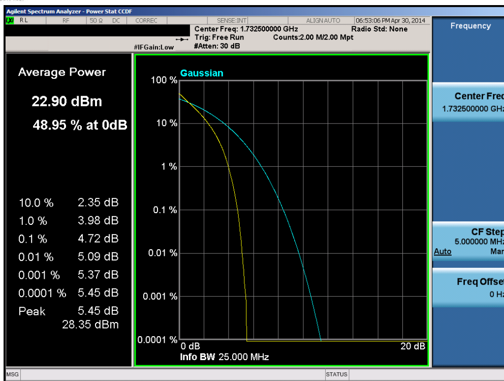
Plot 6-153. PAR Plot (Band 4 – 15.0MHz QPSK – RB Size 75)
