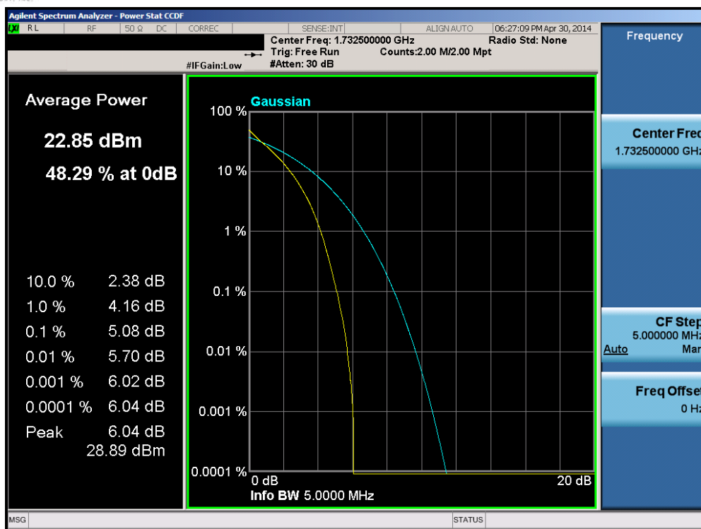
Plot 6-149. PAR Plot (Band 4 – 5.0MHz QPSK – RB Size 25)
