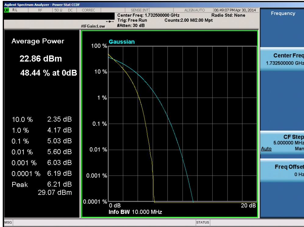
Plot 6-151. PAR Plot (Band 4 – 10.0MHz QPSK – RB Size 50)
