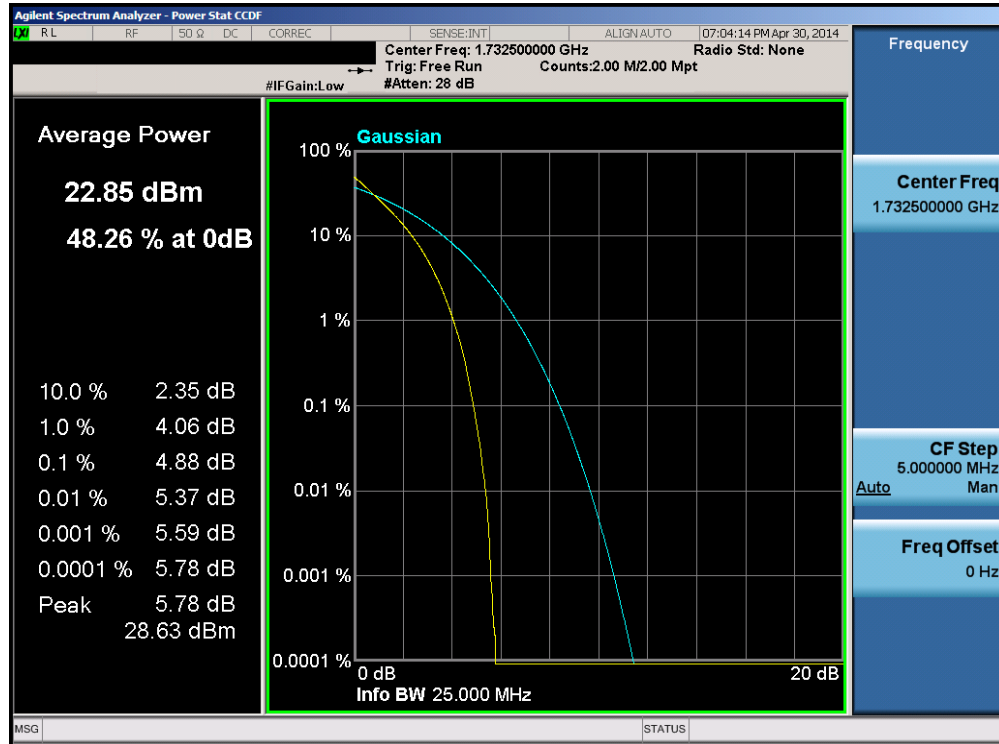
Plot 6-155. PAR Plot (Band 4 – 20.0MHz QPSK – RB Size 100)
