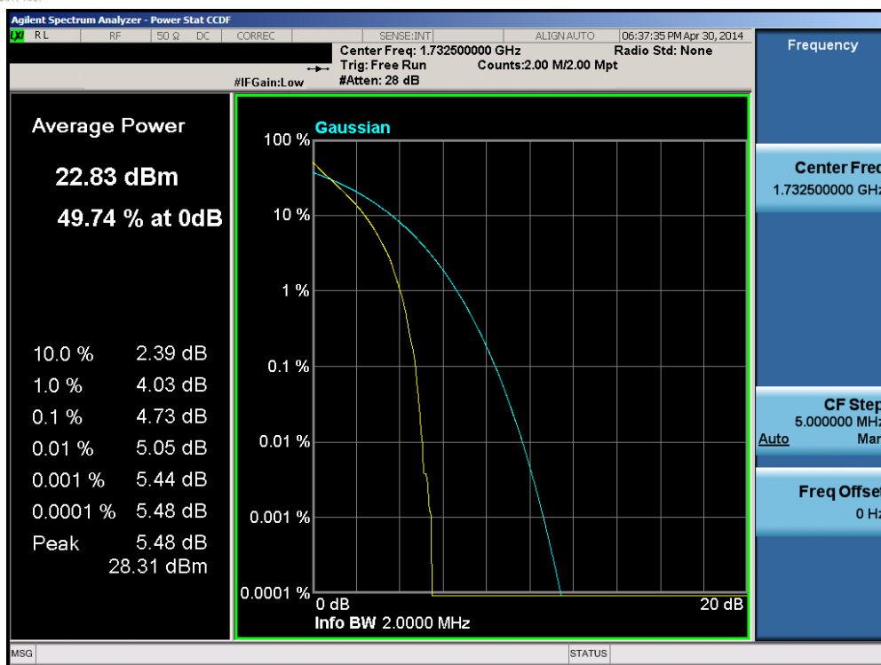
Plot 6-145. PAR Plot (Band 4 – 1.4MHz QPSK – RB Size 6)
