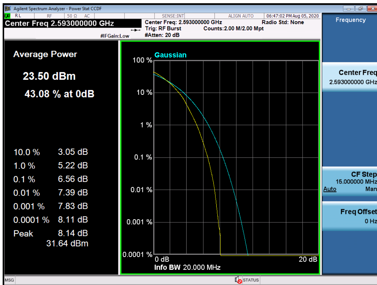
PAR Plot (20M BW_Ch.40620_64QAM_RB100_0) (POWER CLASS 2)
