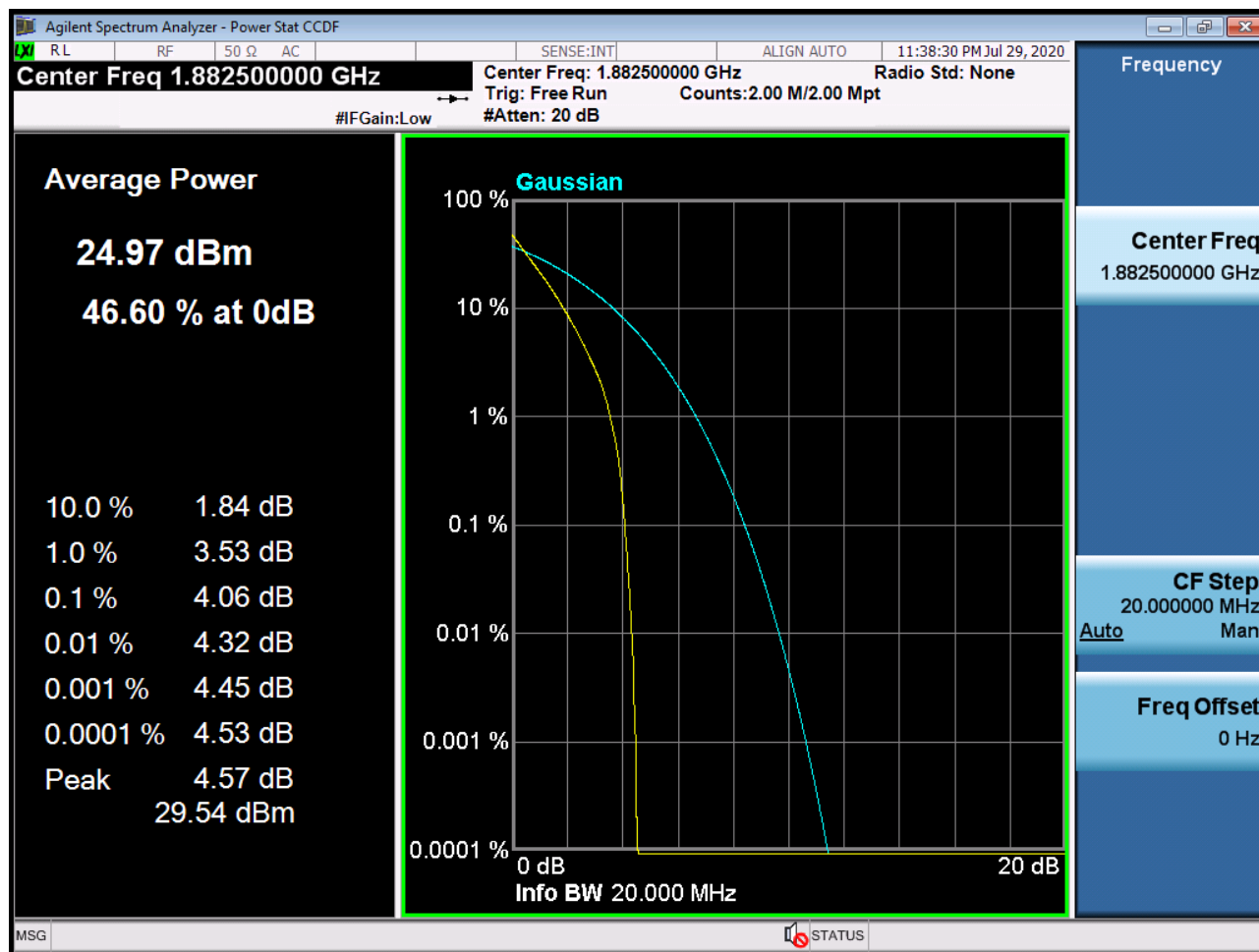
Sub6 n25(2). PAR Plot (20M BW Ch.376500 BPSK RB 100_0)
