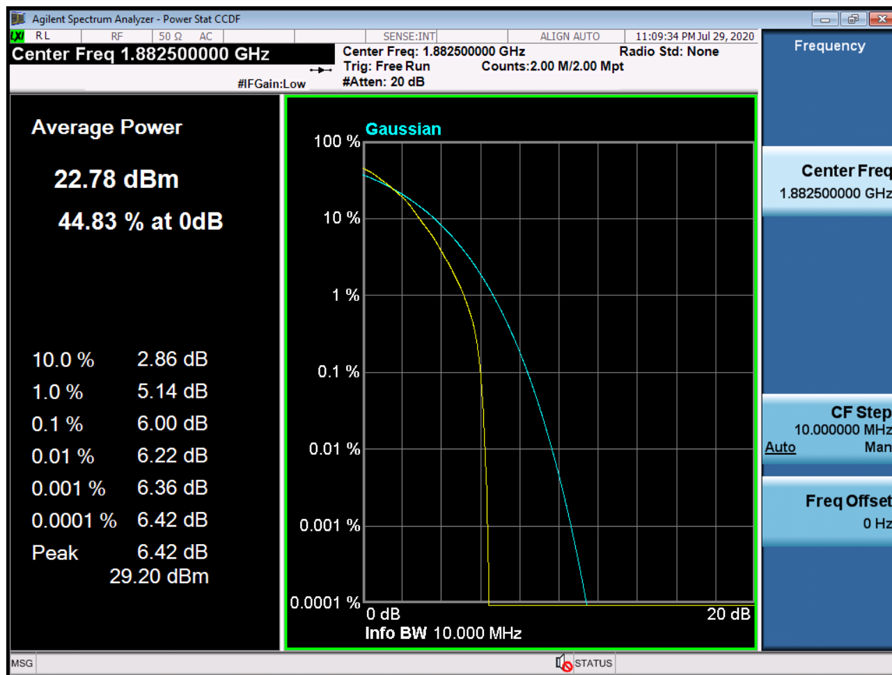
Sub6 n25(2). PAR Plot (10M BW Ch.376500 64QAM RB 50_0)
