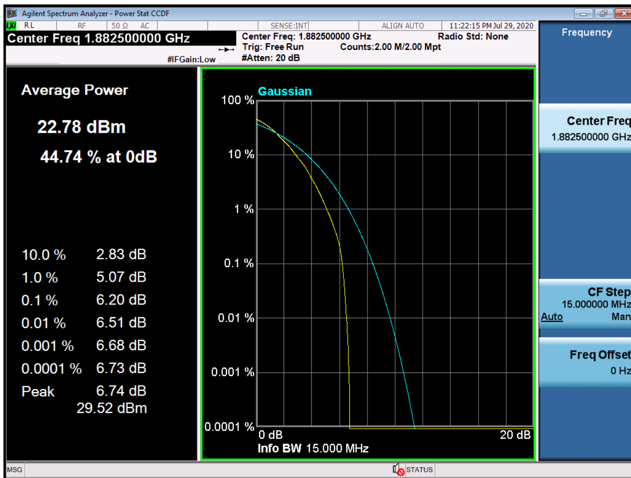
Sub6 n25(2). PAR Plot (15M BW Ch.376500 64QAM RB 75_0)
