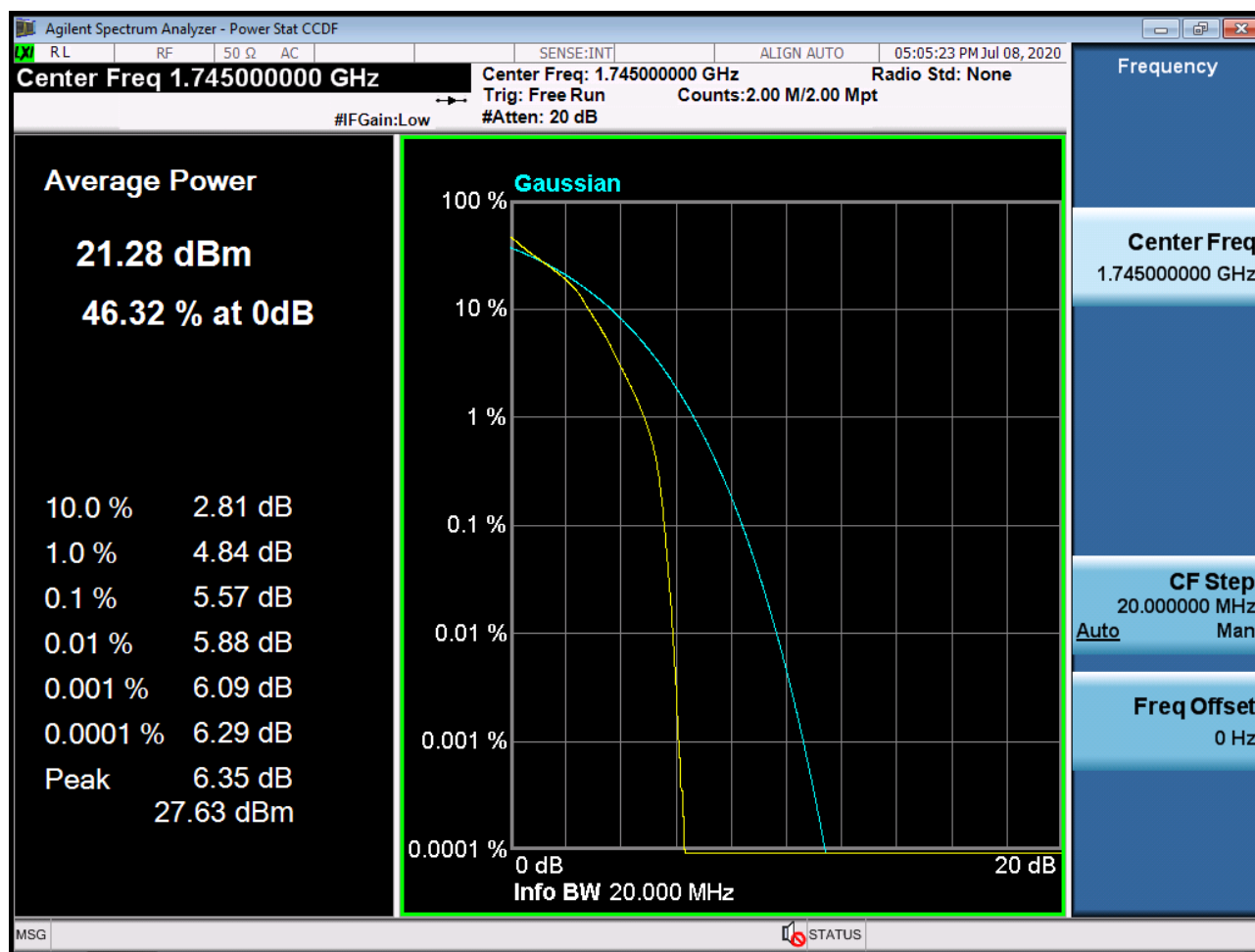
Sub6 n66. PAR Plot (20M BW_Ch.349000_16QAM_RB100_0)
