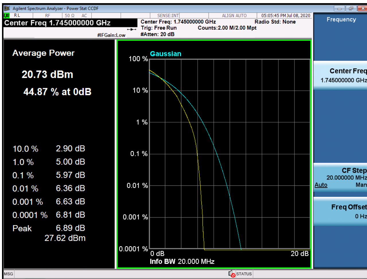
Sub6 n66. PAR Plot (20M BW_Ch.349000_64QAM_RB100_0)
