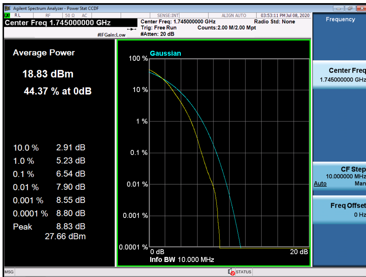
Sub6 n66. PAR Plot (10M BW_Ch.349000_256QAM_RB50_0)
