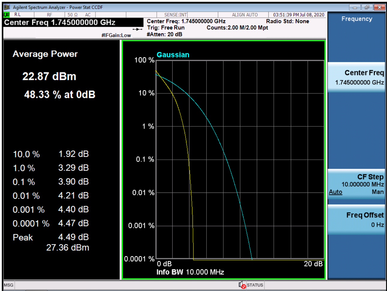
Sub6 n66. PAR Plot (10M BW_Ch.349000_ BPSK_RB50_0)
