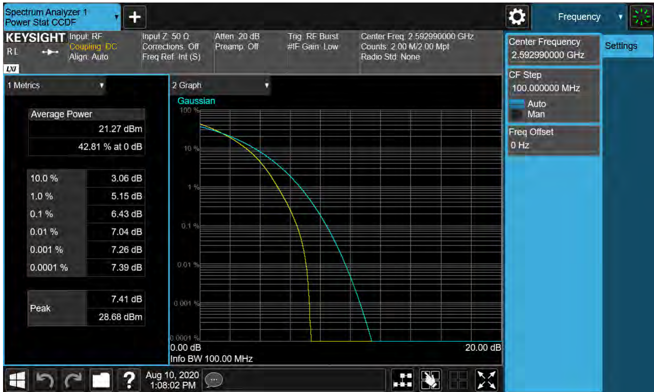
Sub6 n41. PAR Plot (100M BW_Ch.518598_64QAM_RB25_0)
