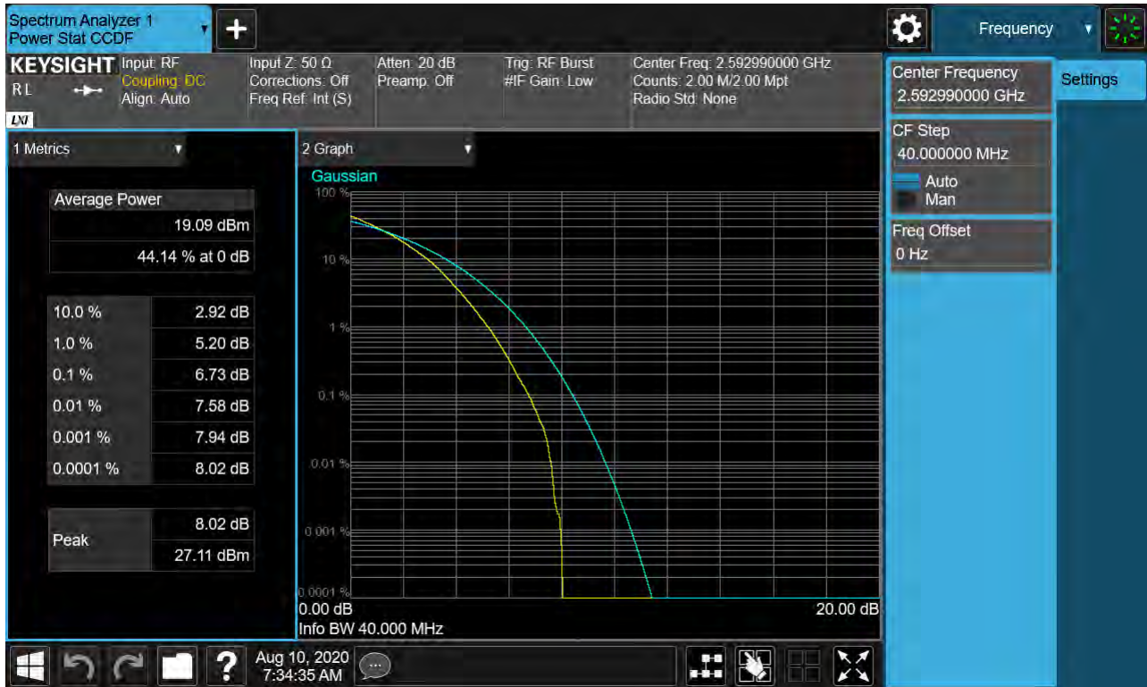
Sub6 n41. PAR Plot (40M BW_Ch.518598_256QAM_RB25_0)
