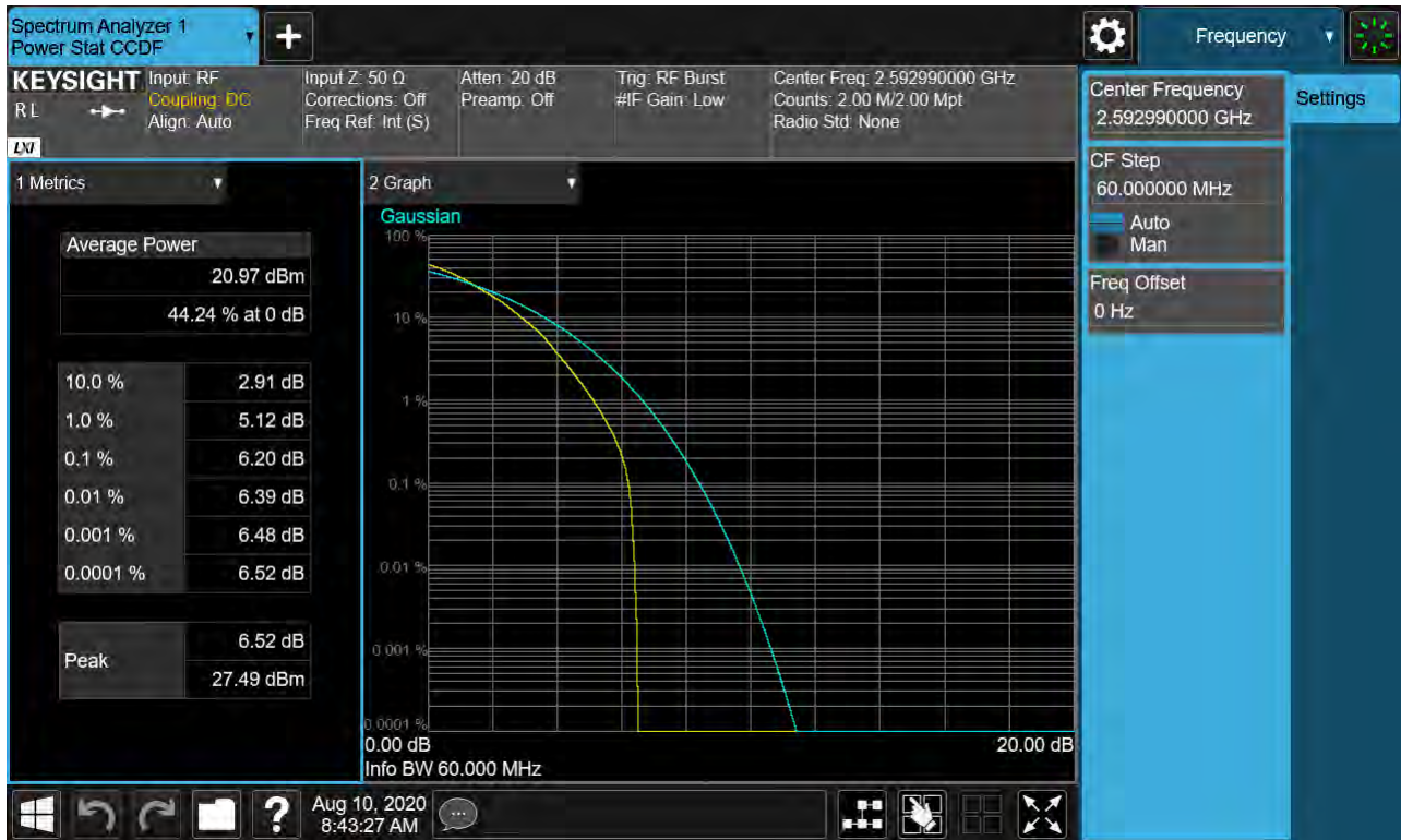
Sub6 n41. PAR Plot (60M BW_Ch.518598_64QAM_RB25_0)
