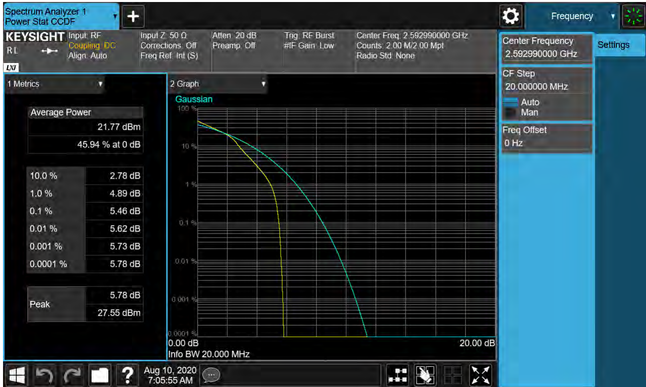
Sub6 n41. PAR Plot (20M BW_Ch.518598_16QAM_RB25_0)
