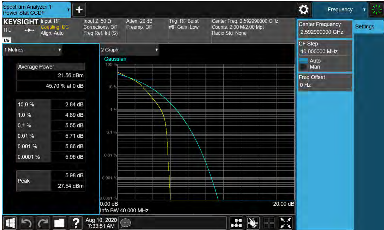
Sub6 n41. PAR Plot (40M BW_Ch.518598_16QAM_RB25_0)
