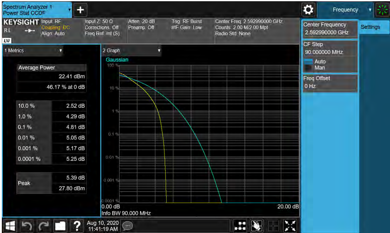
Sub6 n41. PAR Plot (90M BW_Ch.518598_QPSK_RB25_0)
