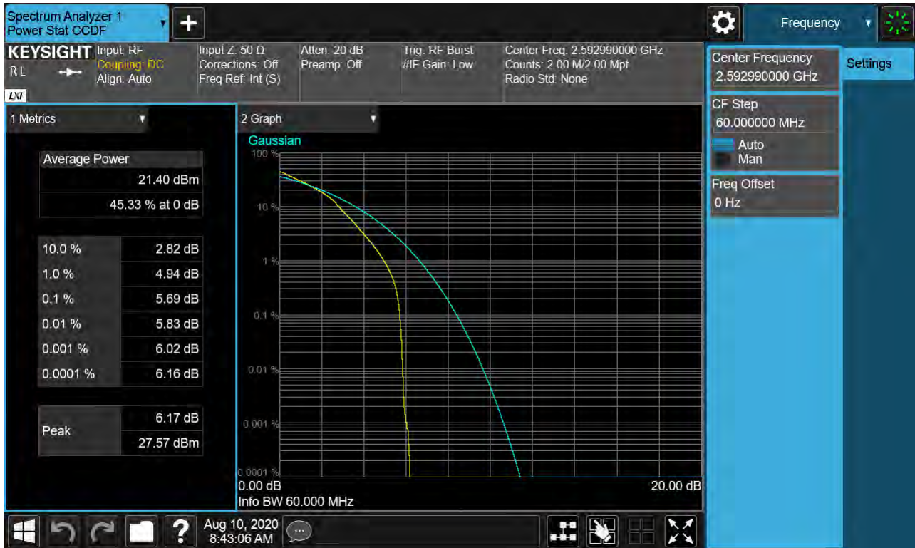
Sub6 n41. PAR Plot (60M BW_Ch.518598_16QAM_RB25_0)
