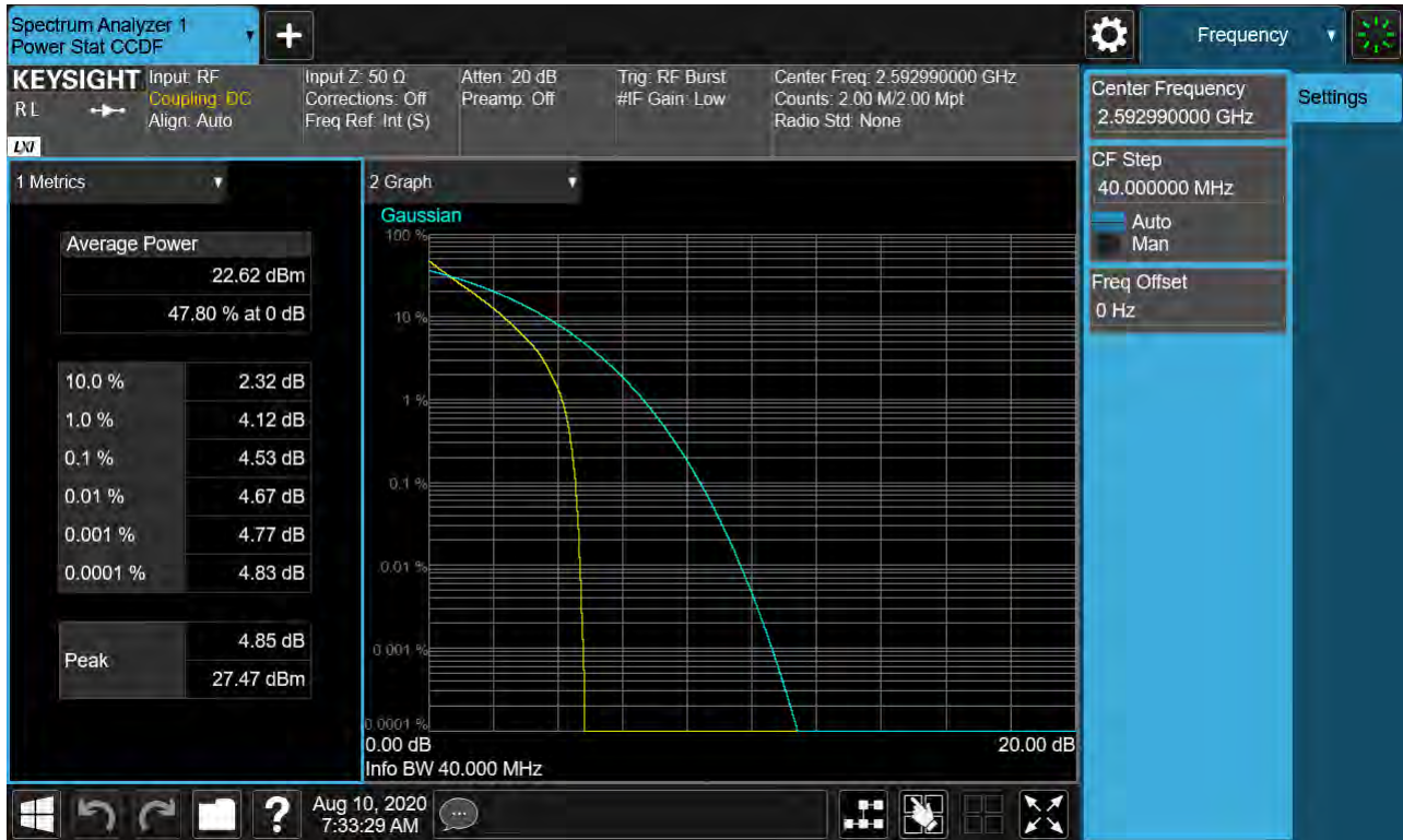
Sub6 n41. PAR Plot (40M BW_Ch.518598_QPSK_RB25_0)
