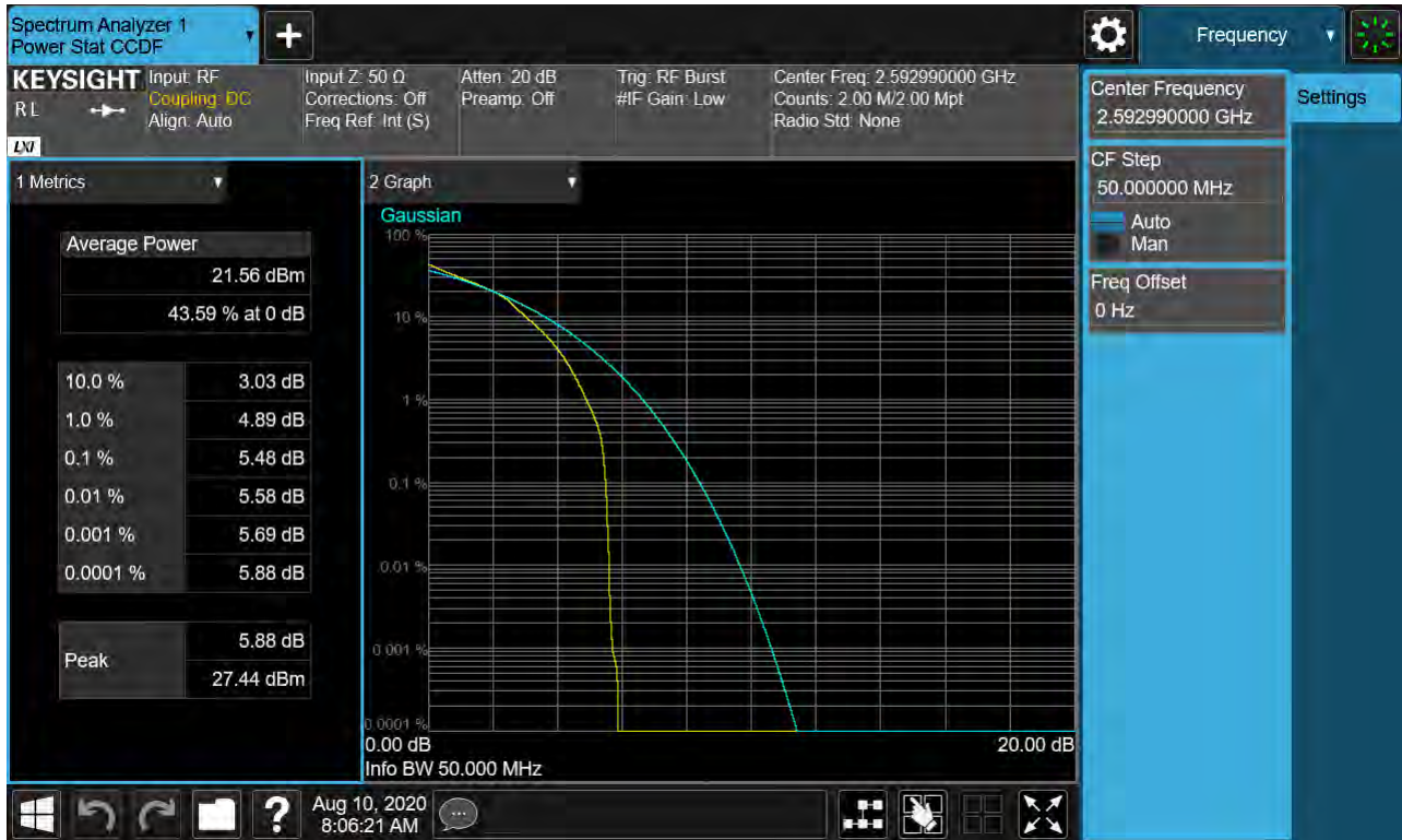
Sub6 n41. PAR Plot (50M BW_Ch.518598_16QAM_RB25_0)
