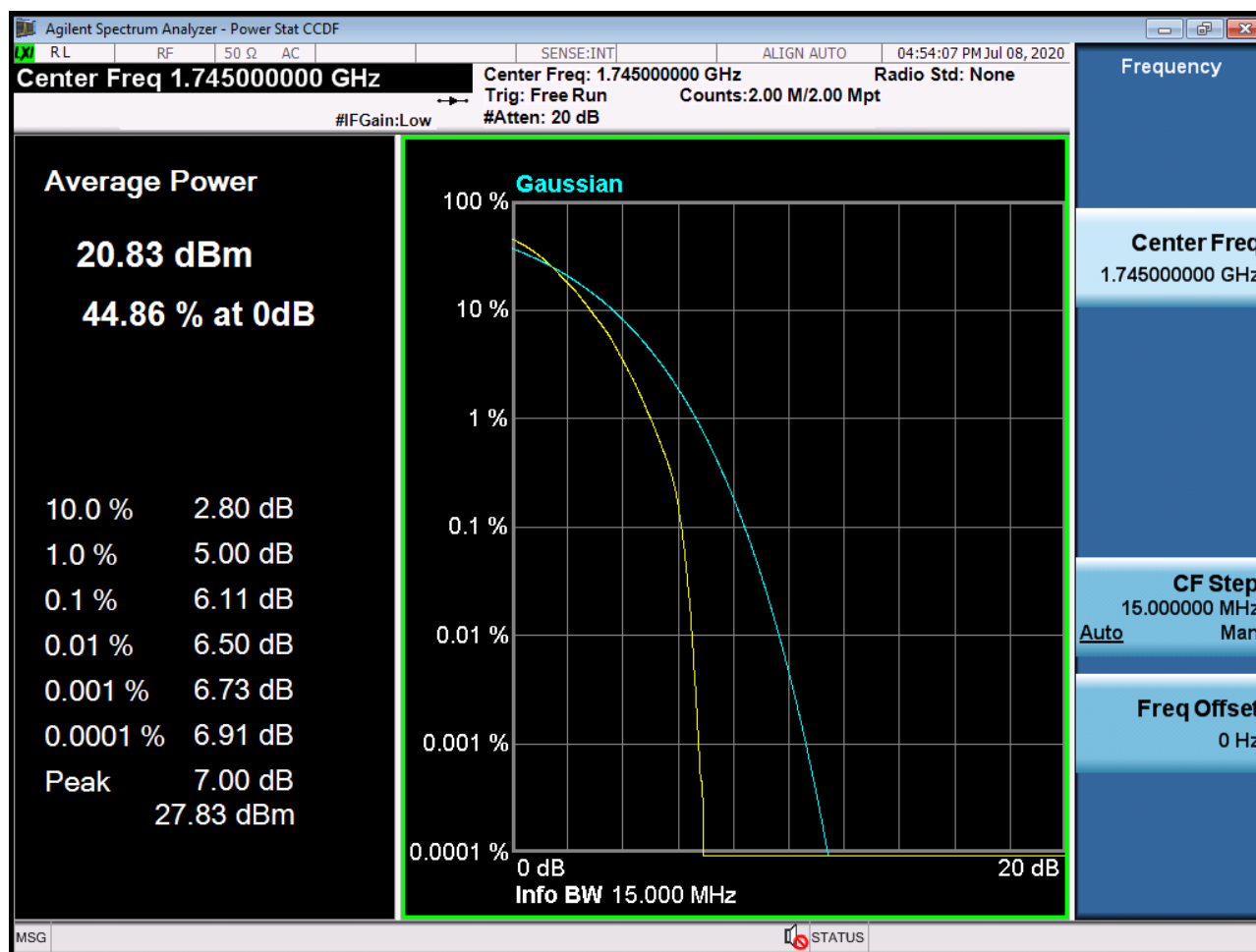
Sub6 n66. PAR Plot (15M BW_Ch.349000_64QAM_RB75_0)
