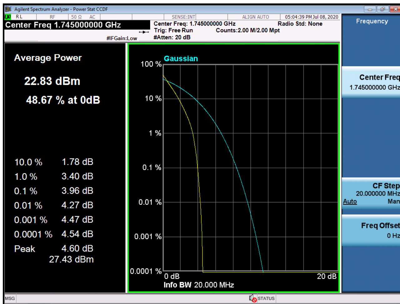
Sub6 n66. PAR Plot (20M BW_Ch.349000_ BPSK_RB100_0)
