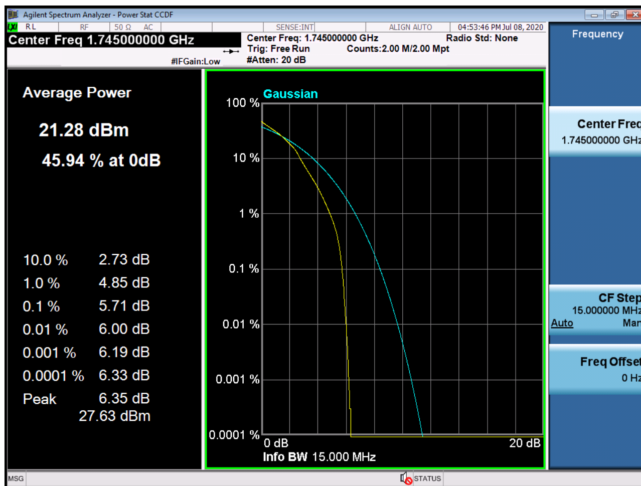
Sub6 n66. PAR Plot (15M BW_Ch.349000_16QAM_RB75_0)
