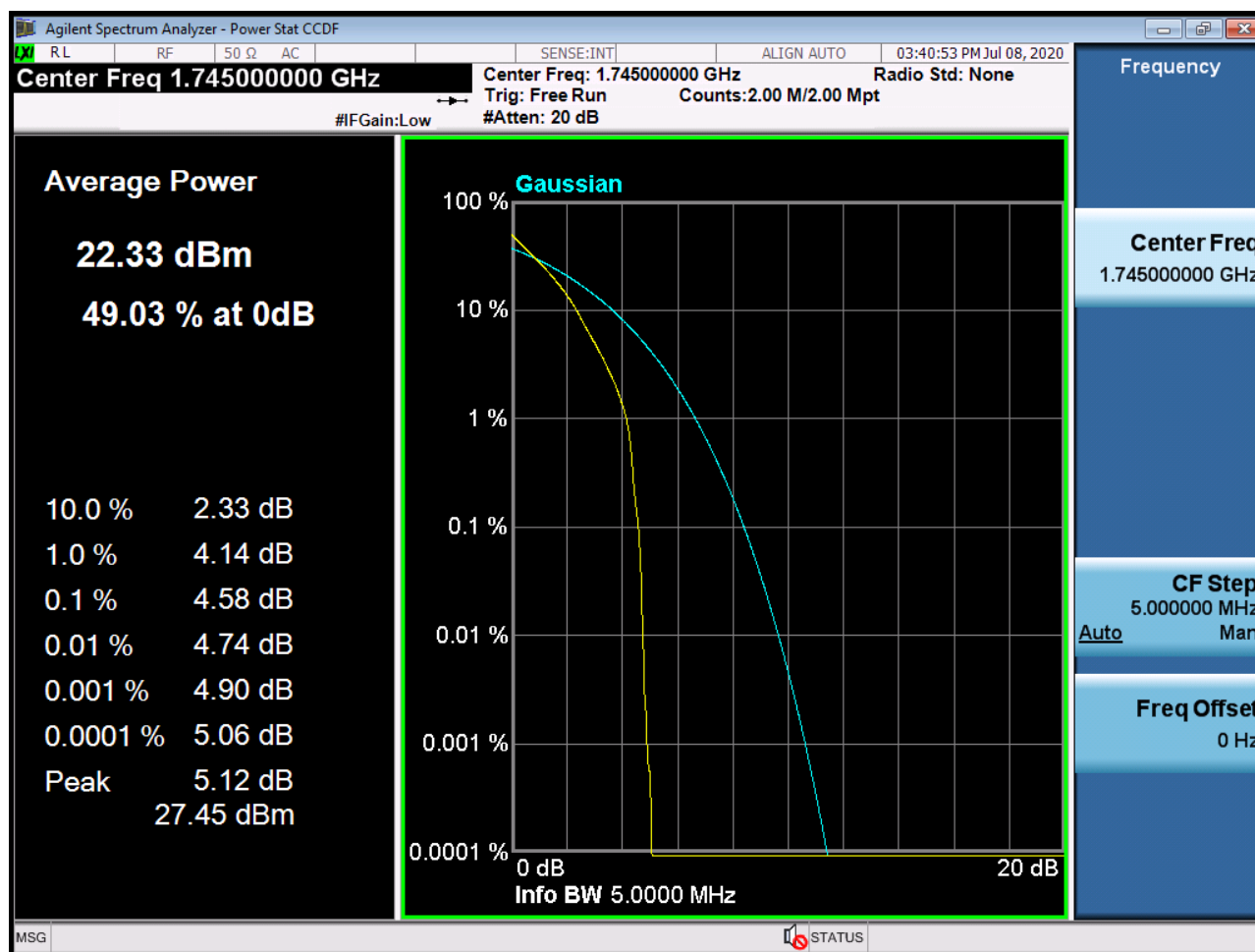
Sub6 n66. PAR Plot (5M BW_Ch.349000_QPSK_RB25_0)
