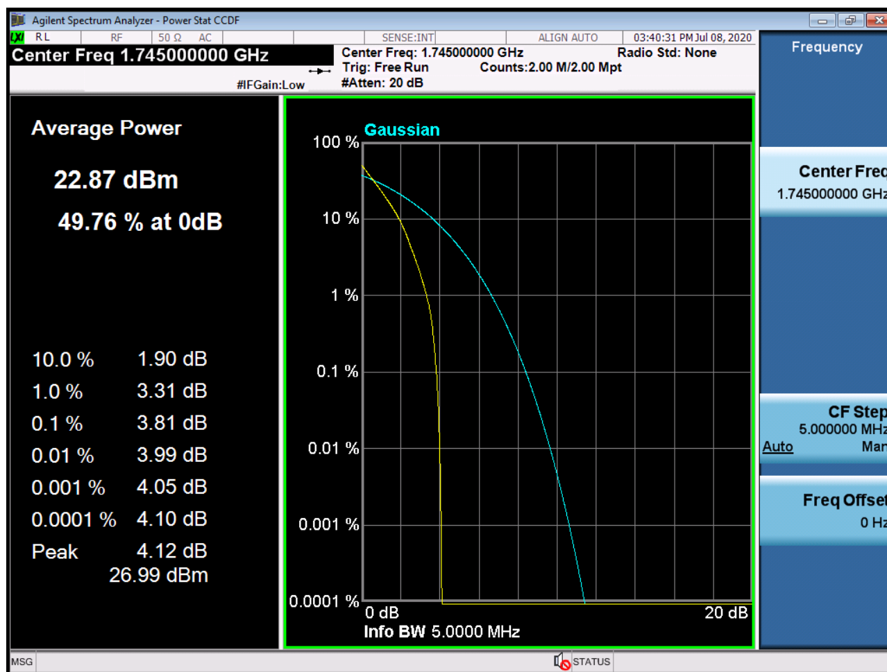
Sub6 n66. PAR Plot (5M BW_Ch.349000_ BPSK_RB25_0)
