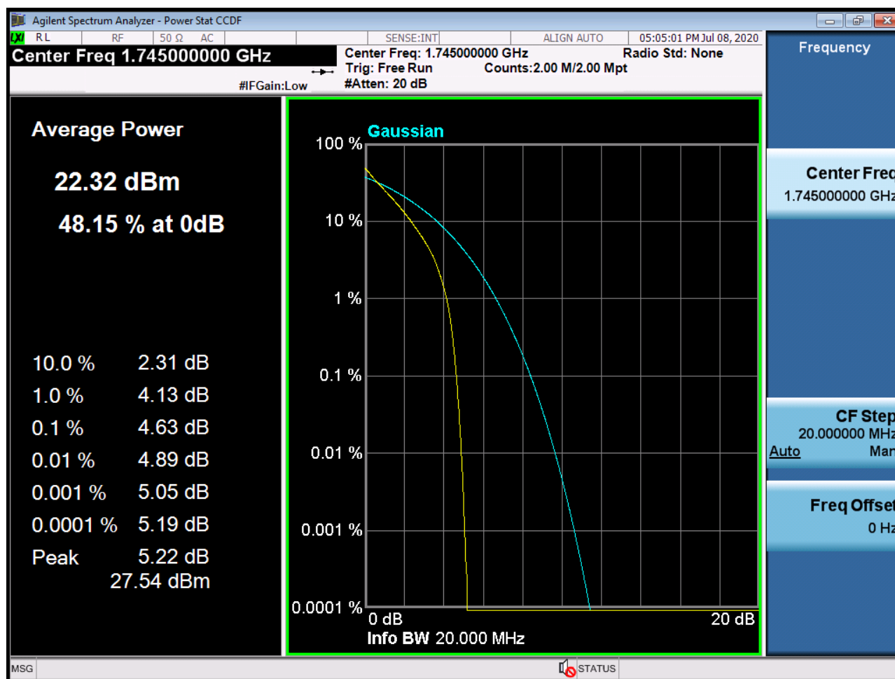
Sub6 n66. PAR Plot (20M BW_Ch.349000_QPSK_RB100_0)
