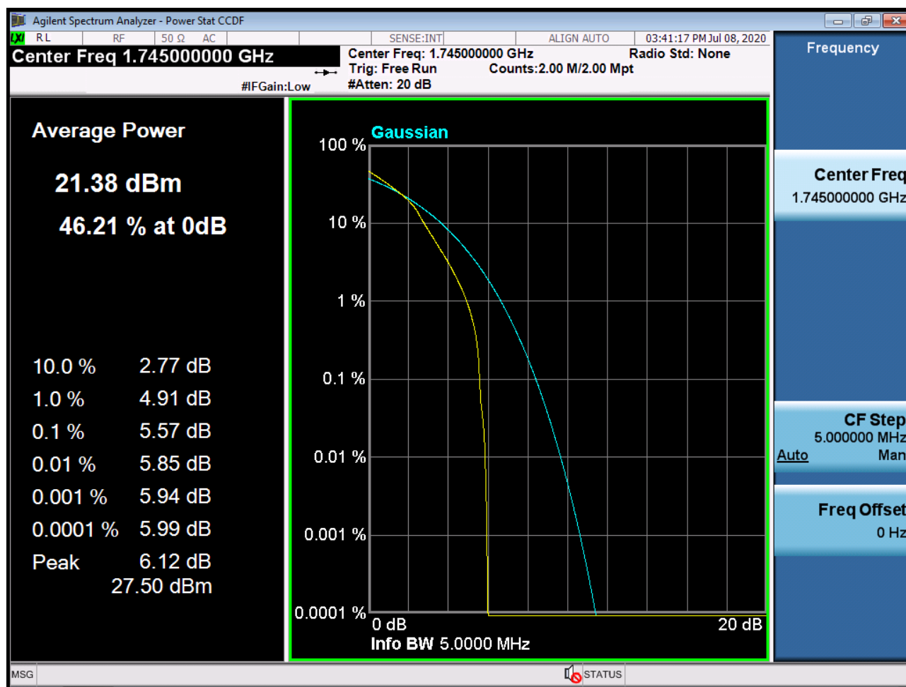
Sub6 n66. PAR Plot (5M BW_Ch.349000_16QAM_RB25_0)
