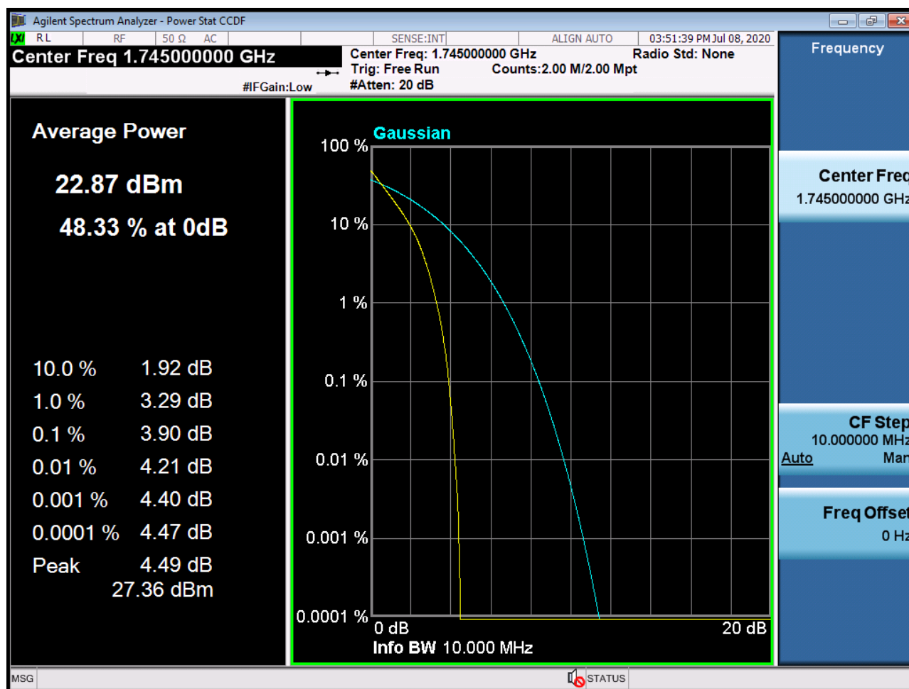
Sub6 n66. PAR Plot (10M BW_Ch.349000_ BPSK_RB50_0)
