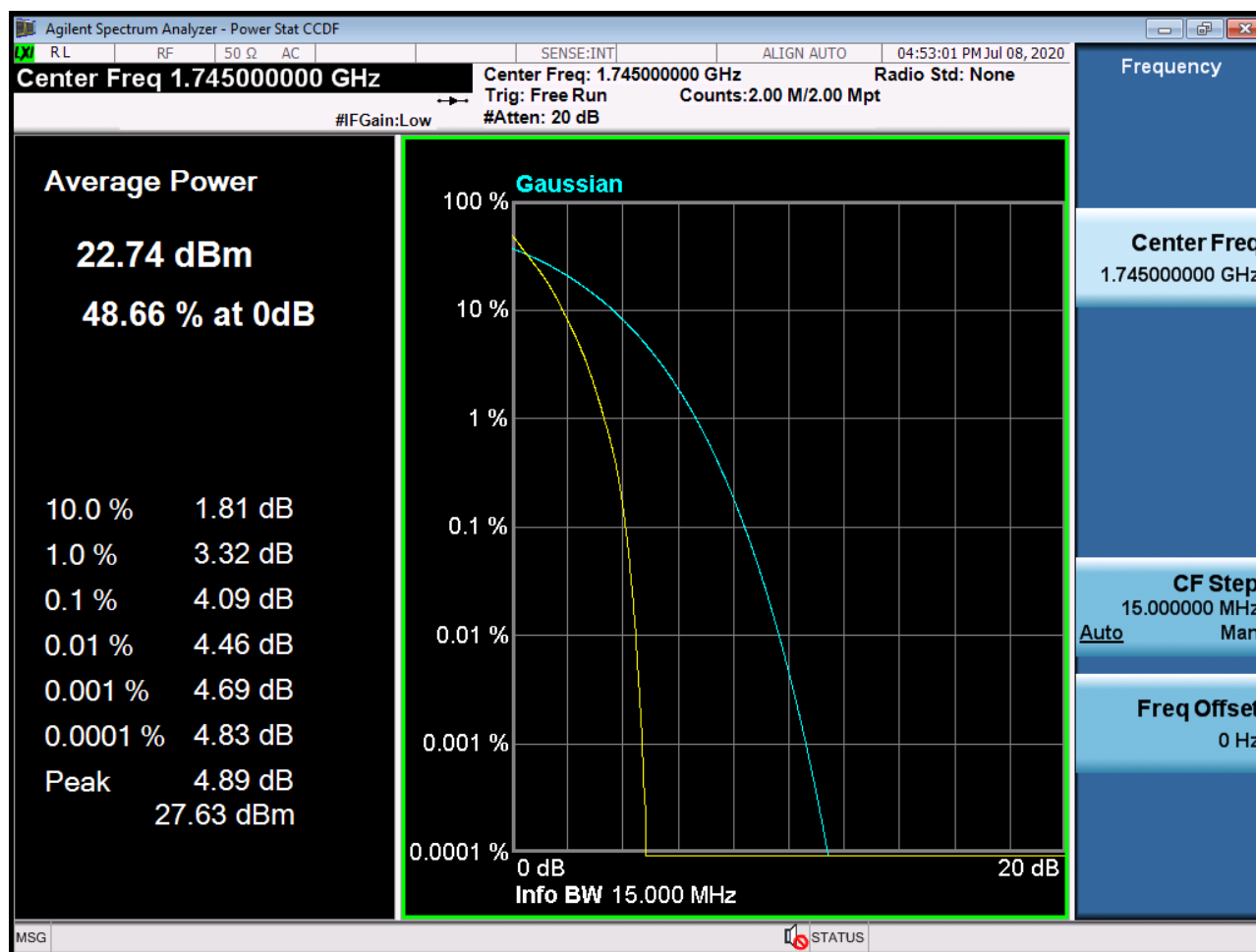
Sub6 n66. PAR Plot (15M BW_Ch.349000_ BPSK_RB75_0)
