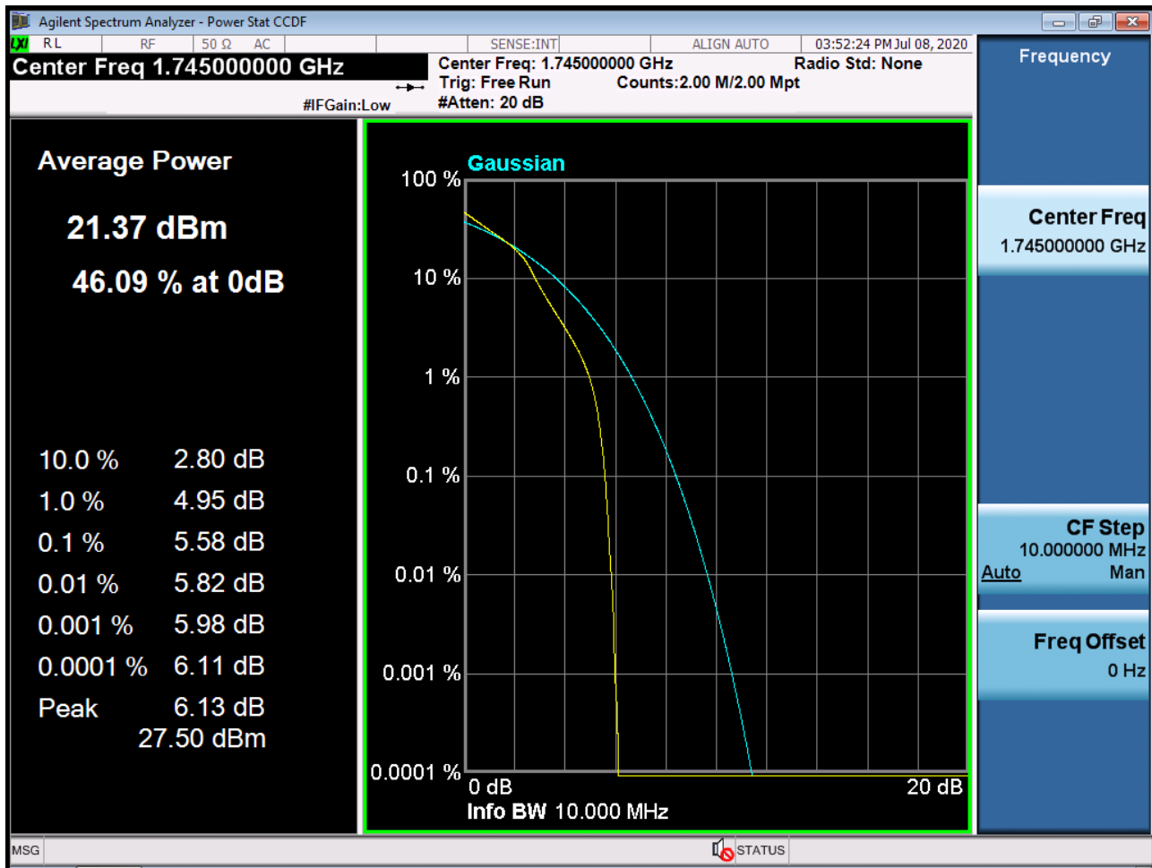
Sub6 n66. PAR Plot (10M BW_Ch.349000_16QAM_RB50_0)
