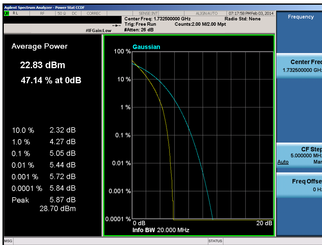
Plot 9-83. PAR Plot (20.0MHz QPSK – RB Size 100)
