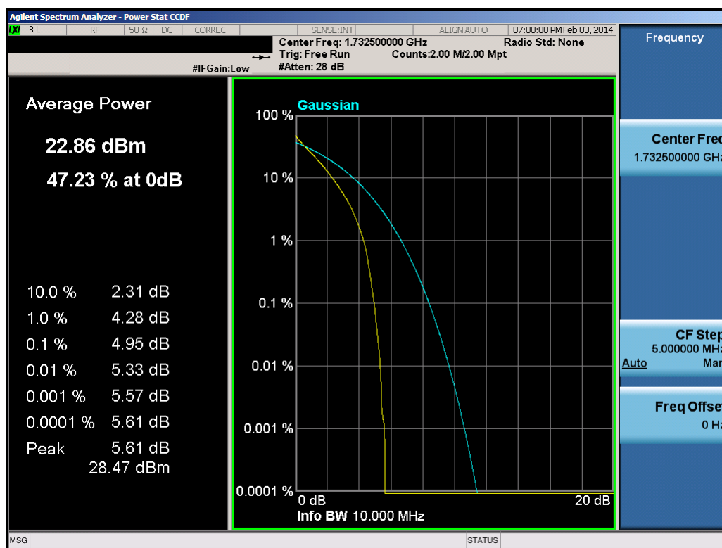
Plot 9-55. PAR Plot (10.0MHz QPSK – RB Size 50)
