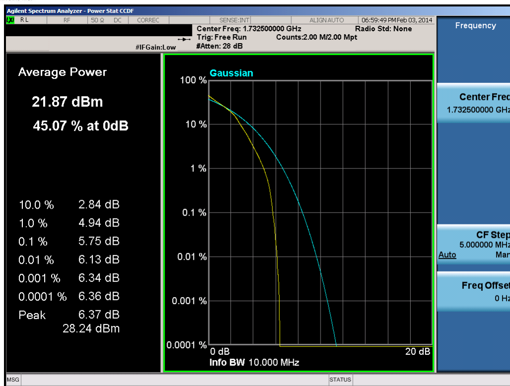
Plot 9-56. PAR Plot (10.0MHz 16-QAM – RB Size 50)
