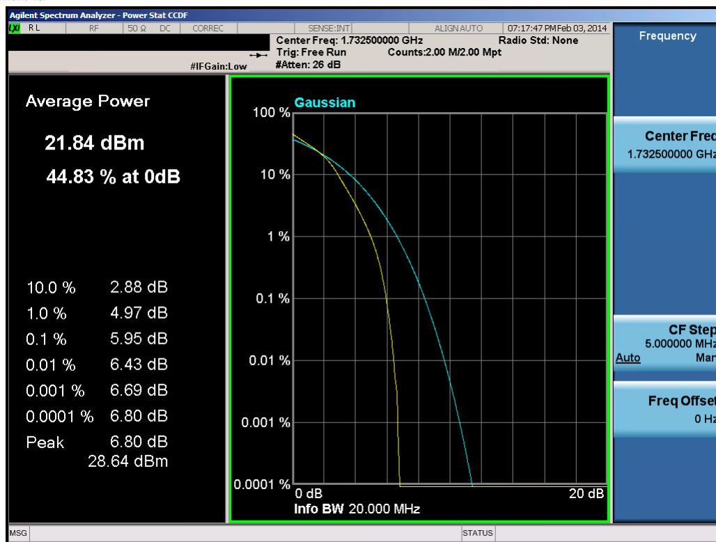
Plot 9-84. PAR Plot (20.0MHz 16-QAM – RB Size 100)
