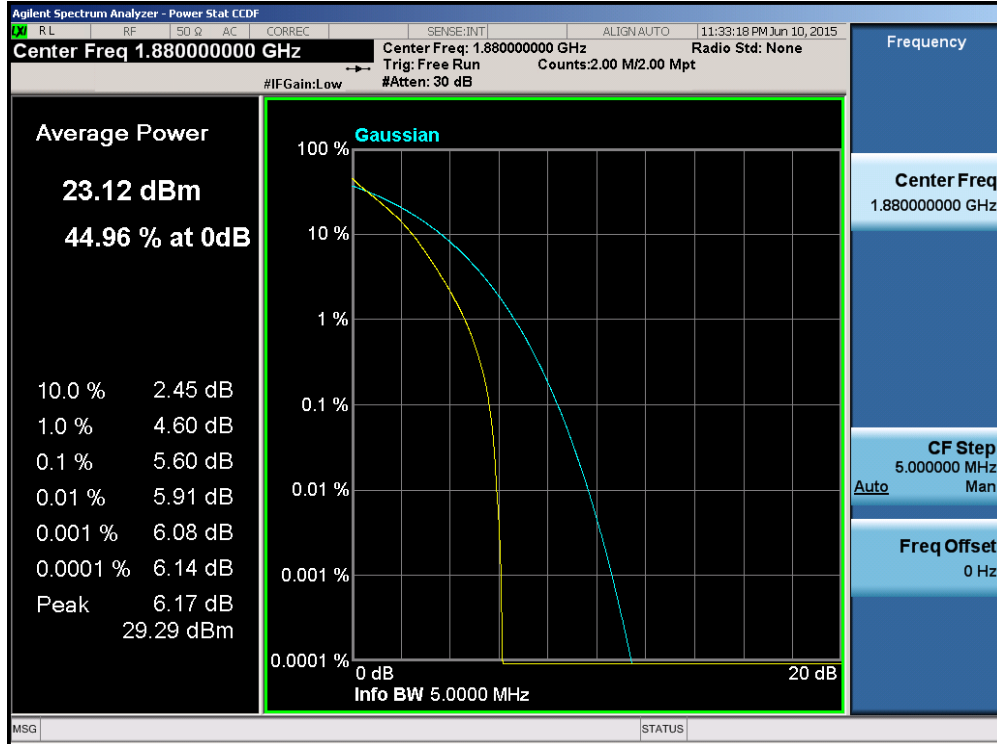
Plot 6-173. PAR Plot (Band 2 – 5.0MHz QPSK – RB Size 25)
