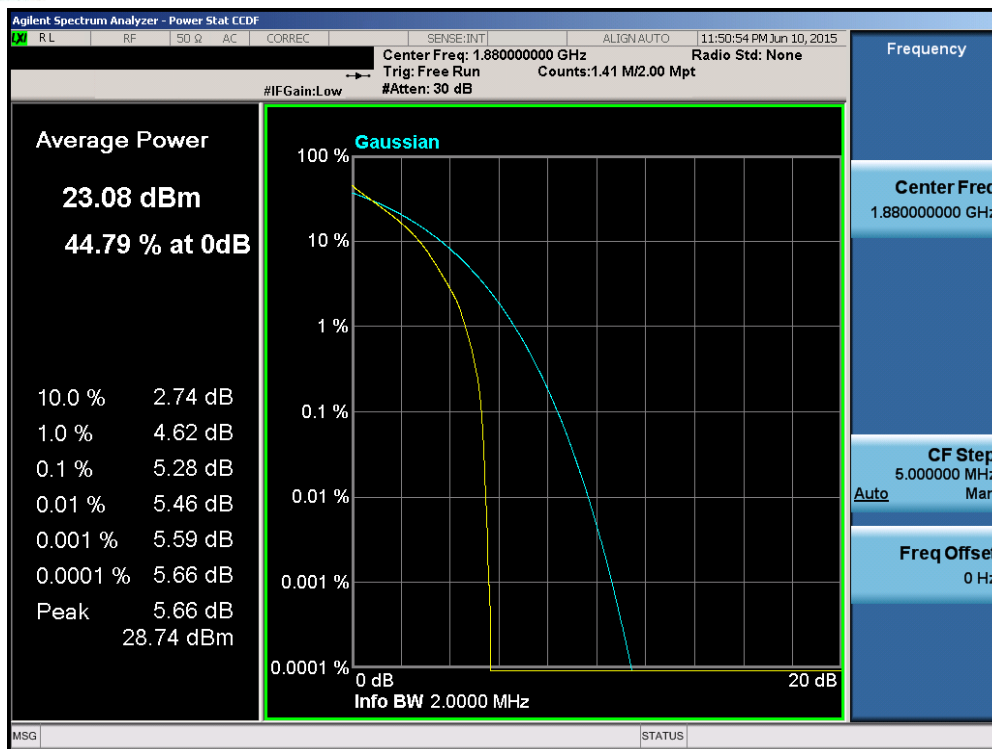
Plot 6-169. PAR Plot (Band 2 – 1.4MHz QPSK – RB Size 6)
