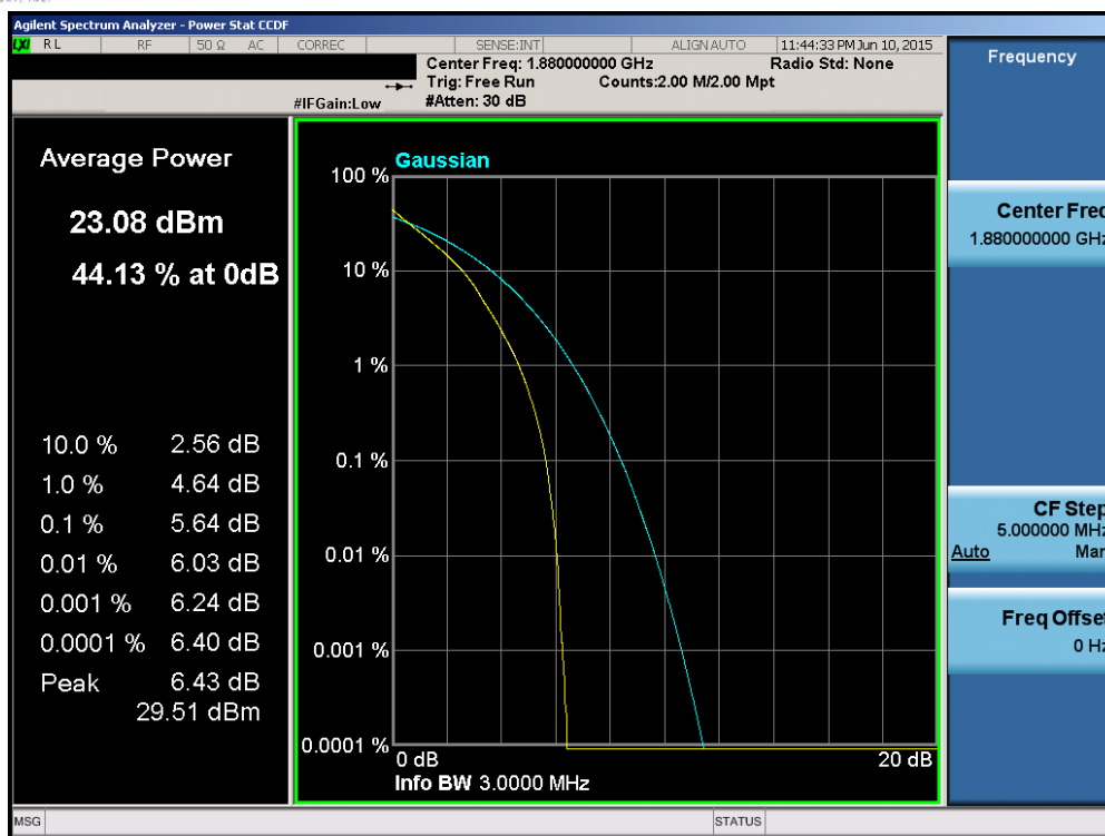
Plot 6-171. PAR Plot (Band 2 – 3.0MHz QPSK – RB Size 15)
