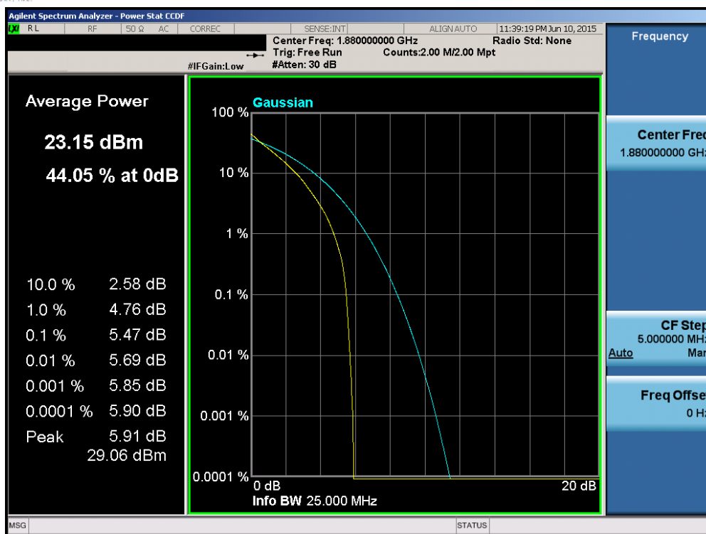
Plot 6-177. PAR Plot (Band 2 – 15.0MHz QPSK – RB Size 75)
