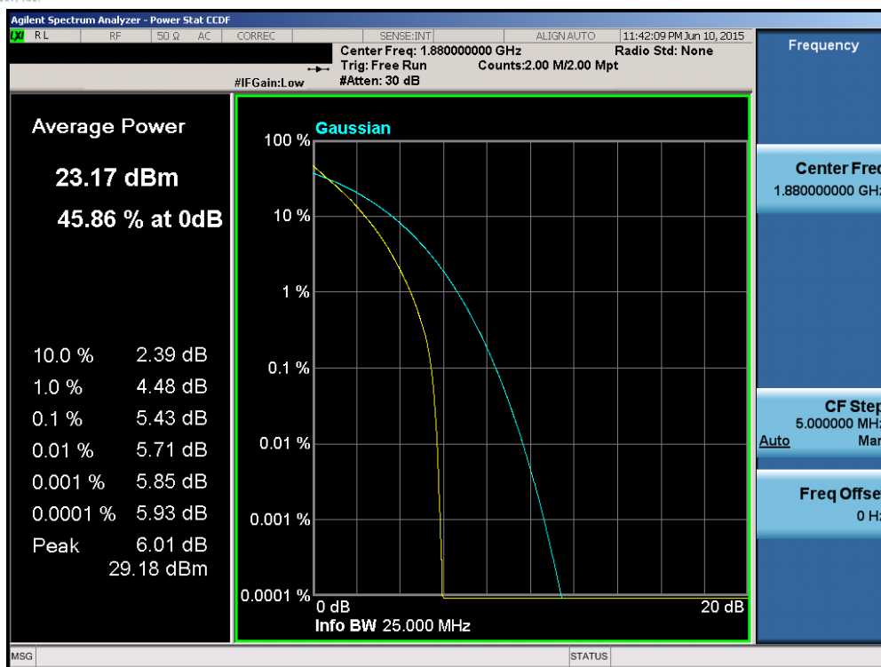
Plot 6-179. PAR Plot (Band 2 – 20.0MHz QPSK – RB Size 100)
