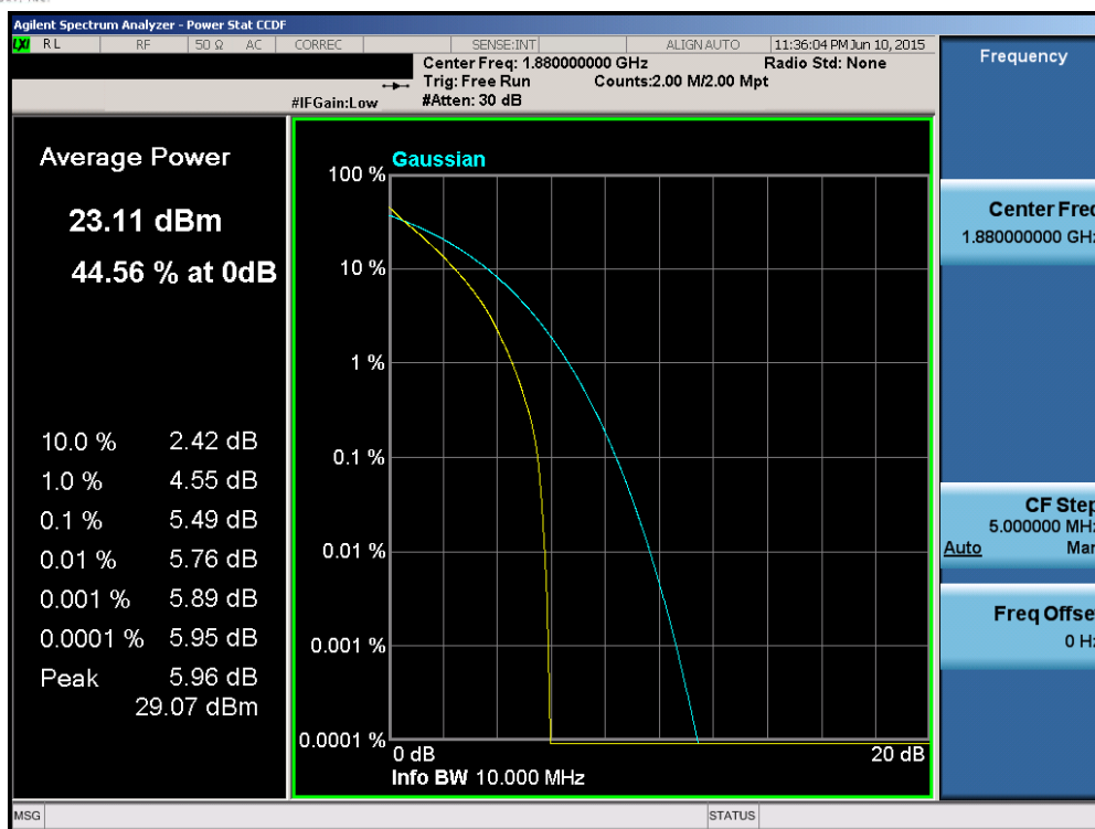
Plot 6-175. PAR Plot (Band 2 – 10.0MHz QPSK – RB Size 50)
