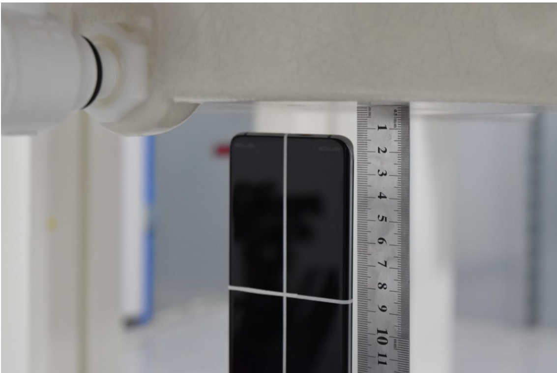
Edge 3 (13 mm)
