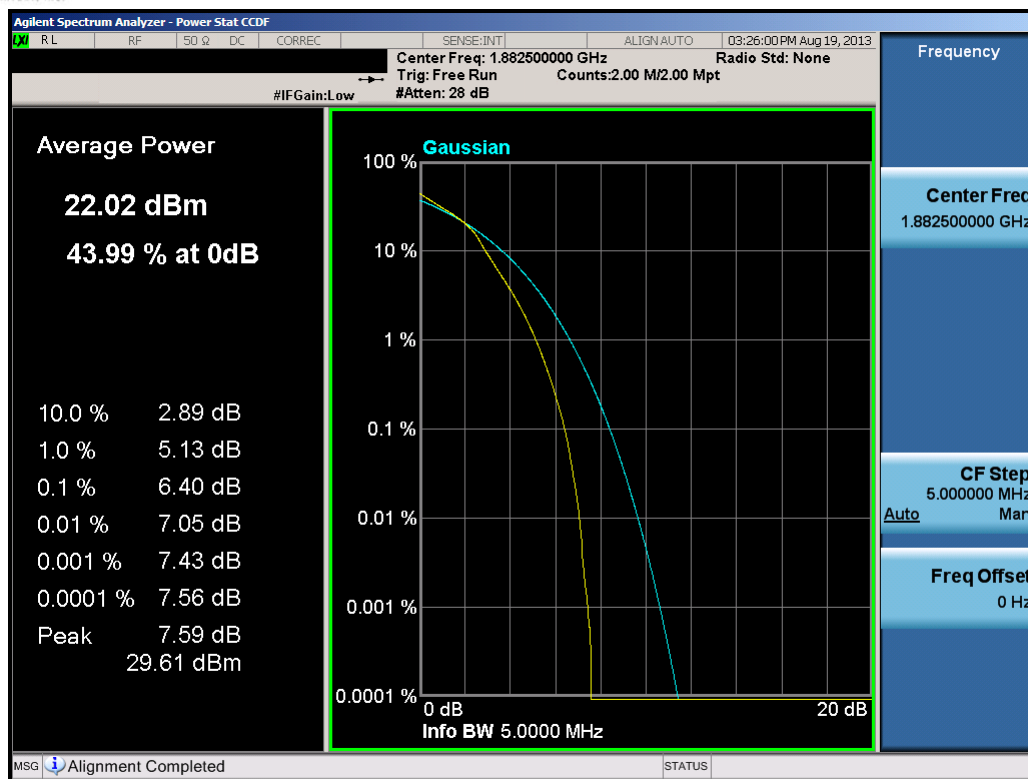
Plot 7-14. PAR Plot (5.0MHz 16-QAM - RB Size 25)
