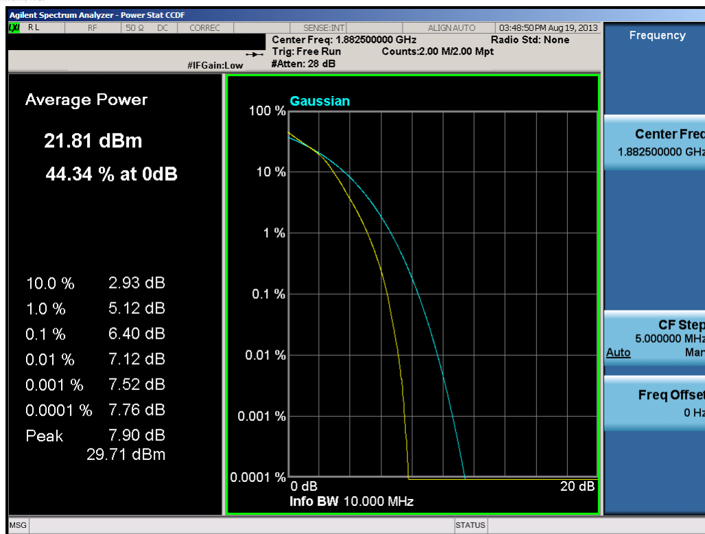
Plot 7-28. PAR Plot (10.0MHz 16-QAM – RB Size 50)
