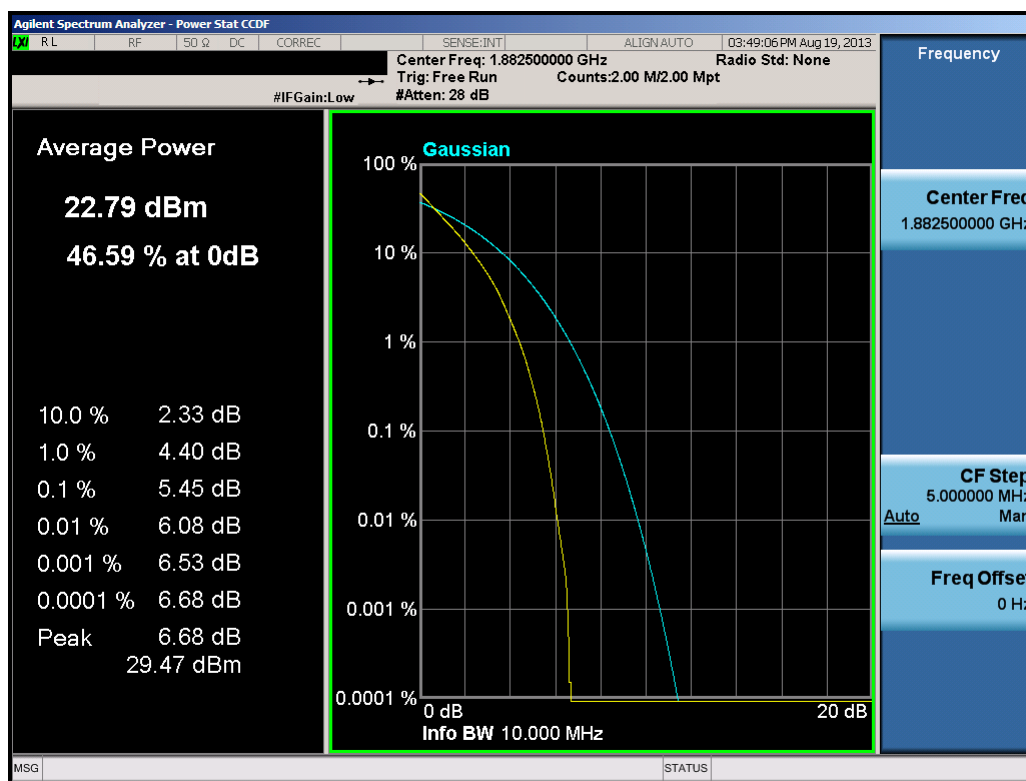
Plot 7-27. PAR Plot (10.0MHz QPSK – RB Size 50)
