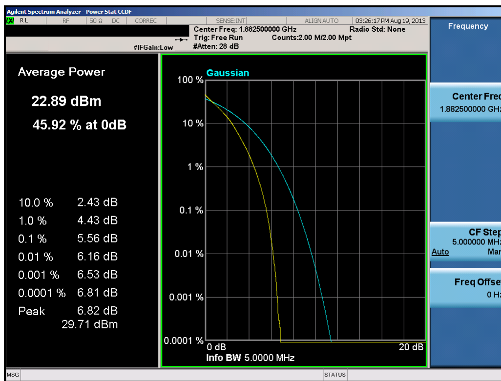
Plot 7-13. PAR Plot (5.0MHz QPSK – RB Size 25)
