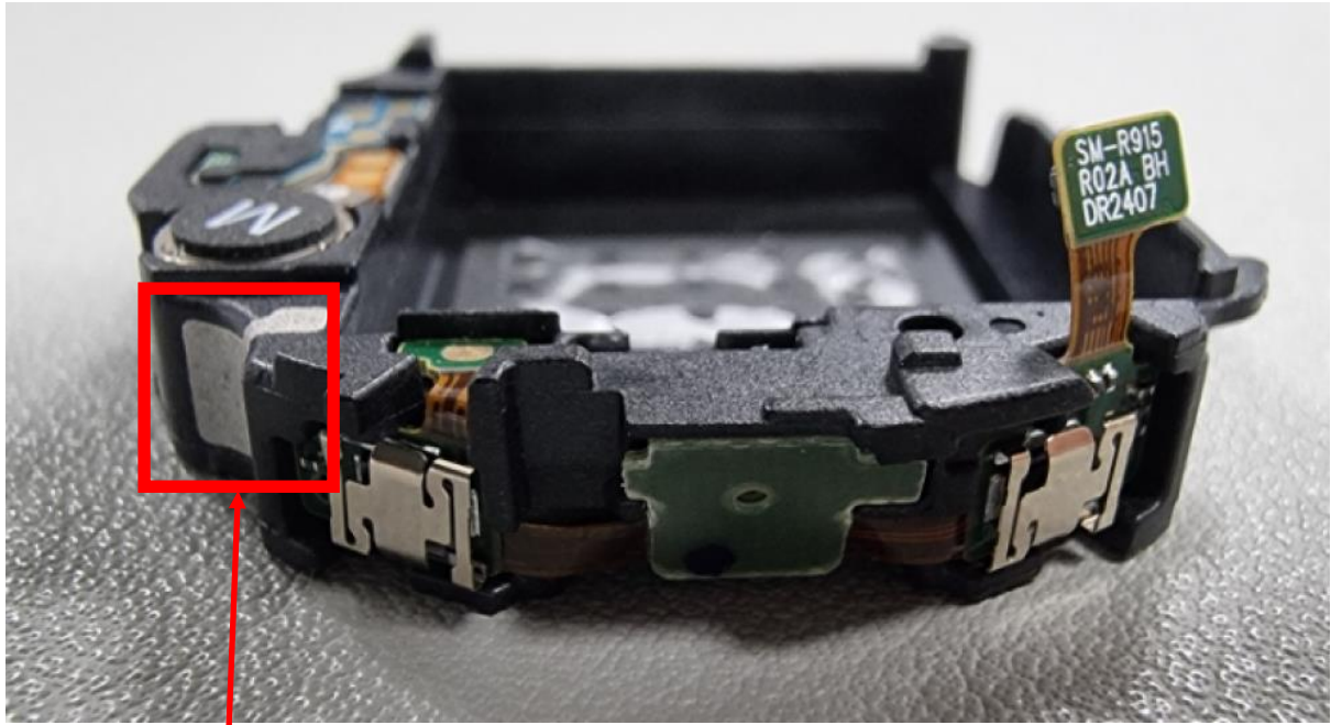
BT/WIFI Ant
