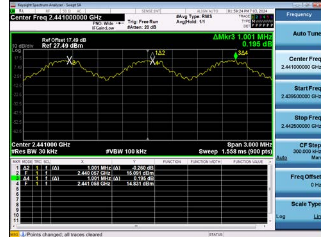
ANT. 1 \pi/4 DQPSK : Channel Separation
