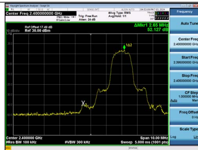
ANT.2 \pi /4DQPSK Band Edge(CH.0)
