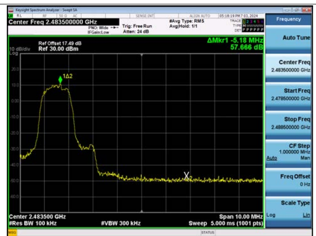
ANT.2 8DPSK Band Edge(CH.78)
