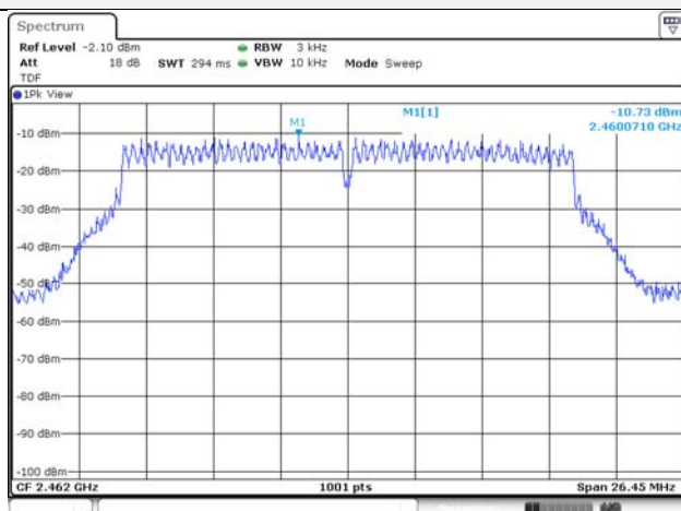
802.11ac VHT20 / 2 462 MHz
