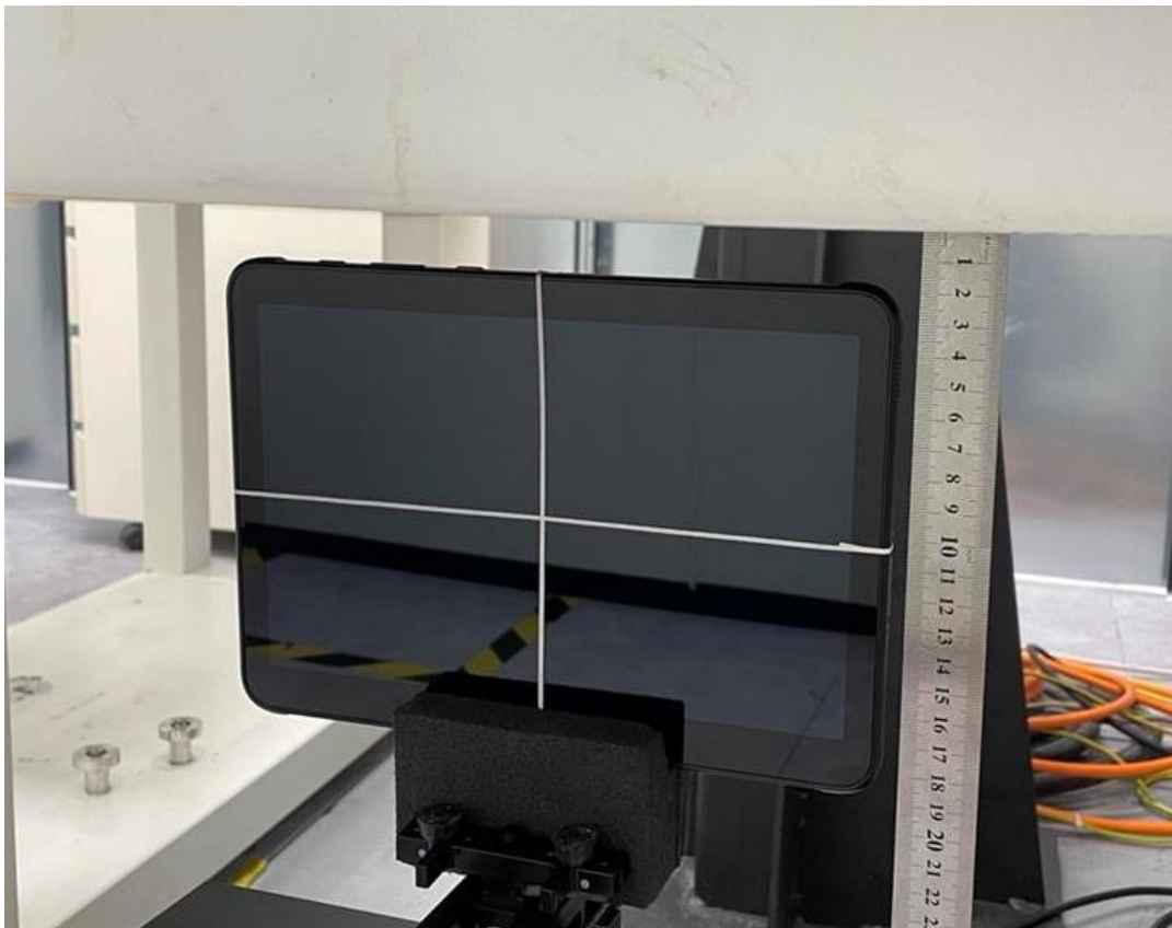
Edge 1 (16mm)
