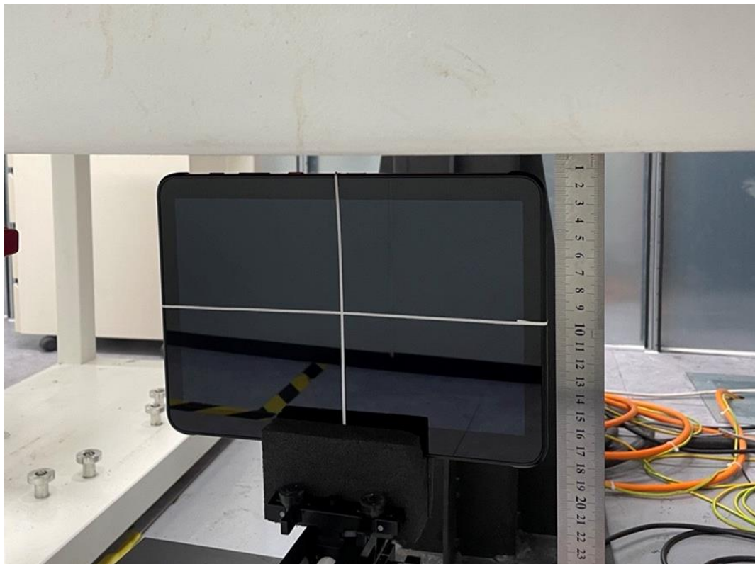
Edge 1 (11mm)
