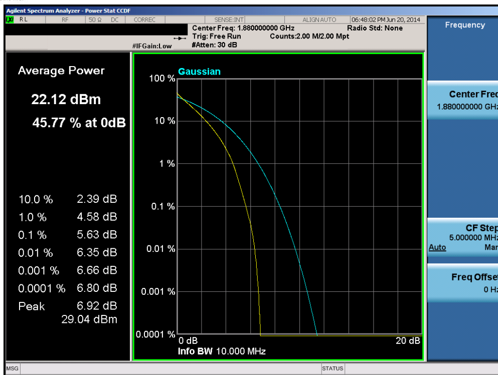
Plot 6-77. PAR Plot (Band 2 – 10.0MHz QPSK – RB Size 50)
