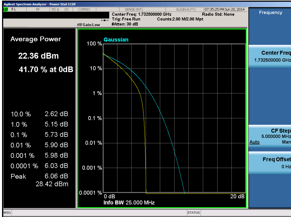
Plot 6-71. PAR Plot (Band 4 – 15.0MHz QPSK – RB Size 75)
