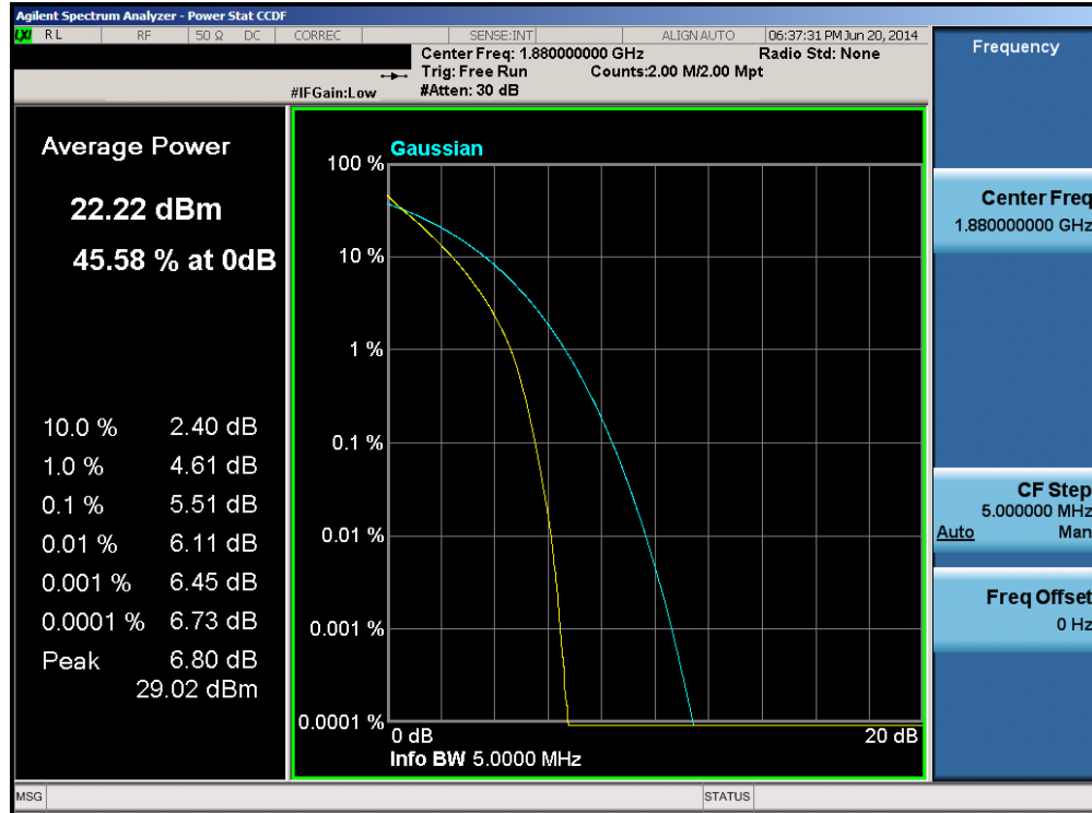
Plot 6-75. PAR Plot (Band 2 – 5.0MHz QPSK – RB Size 25)
