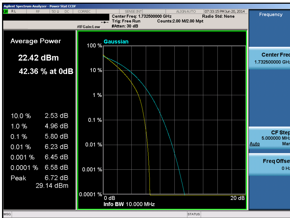
Plot 6-69. PAR Plot (Band 4 – 10.0MHz QPSK – RB Size 50)
