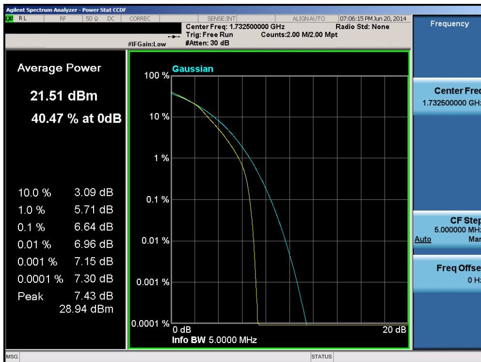
Plot 6-68. PAR Plot (Band 4 – 5.0MHz 16-QAM – RB Size 25)
