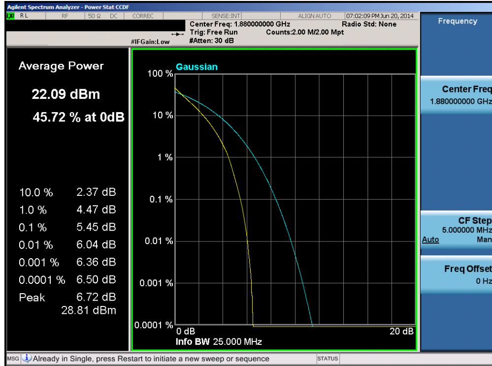
Plot 6-81. PAR Plot (Band 2 – 20.0MHz QPSK – RB Size 100)
