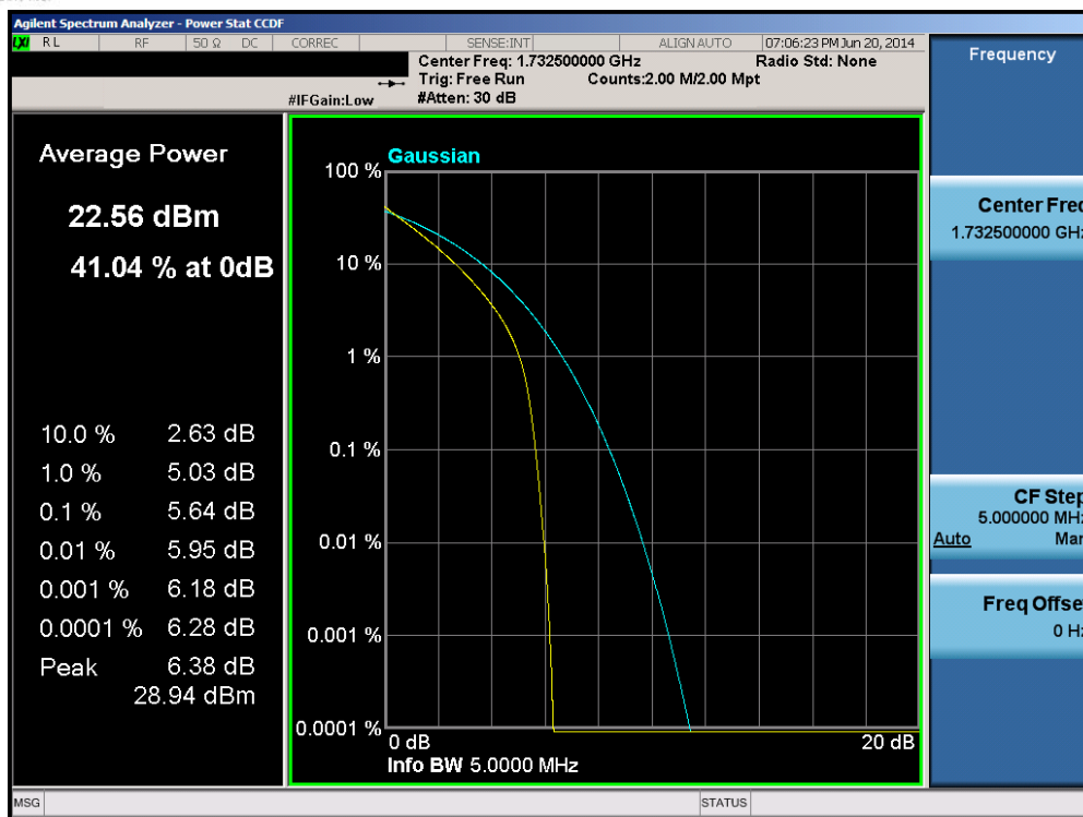
Plot 6-67. PAR Plot (Band 4 – 5.0MHz QPSK – RB Size 25)
