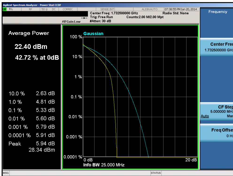
Plot 6-73. PAR Plot (Band 4 – 20.0MHz QPSK – RB Size 100)
