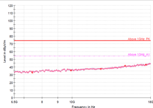
6.5 GHz - 18 GHz
