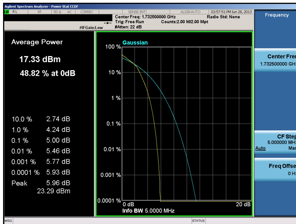
Plot 8-14. PAR Plot (5.0MHz 16-QAM – RB Size 25)
