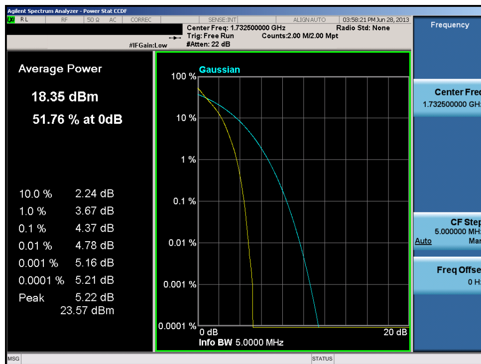
Plot 8-13. PAR Plot (5.0MHz QPSK – RB Size 25)
