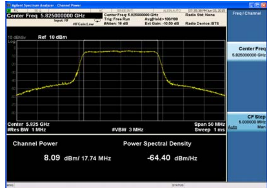
Ant : A3_802.11n_HT20 (2)
