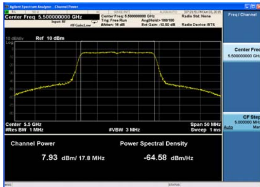
Ant : A3_802.11n_HT20 (1)
