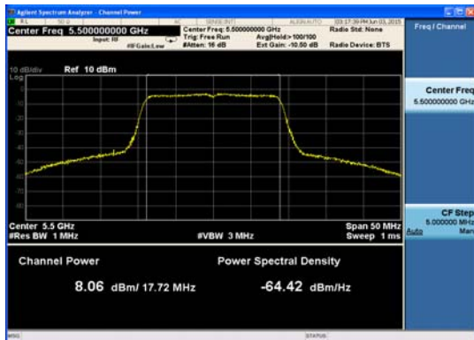
Ant : A2_802.11n_HT20 (1)
