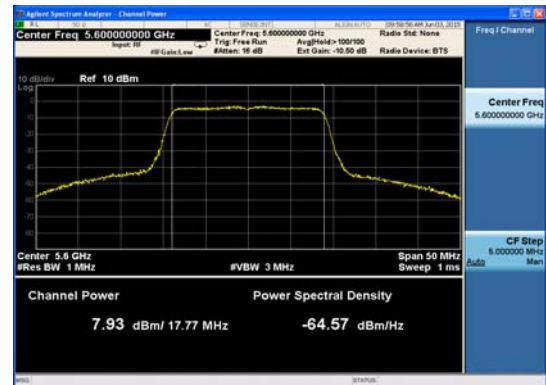
Ant : A1_802.11n_HT20 (1)
