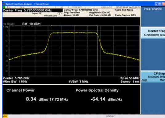
Ant : A1_802.11n_HT20 (2)
