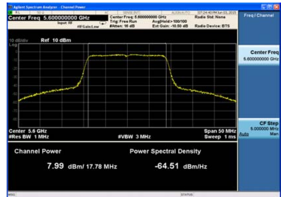
Ant : A3_802.11n_HT20 (1)
