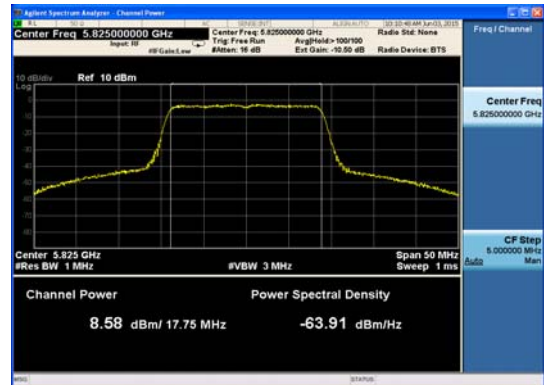
Ant : A1_802.11n_HT20 (2)
