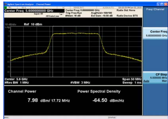
Ant : A2_802.11n_HT20 (1)
