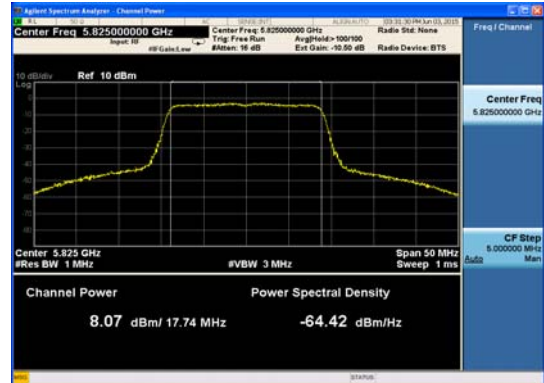
Ant : A2_802.11n_HT20 (2)
