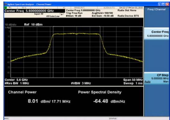
Ant : A2_802.11ac_VHT20 (1)
