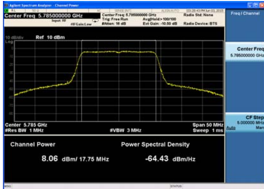
Ant : A2_802.11n_HT20 (2)
