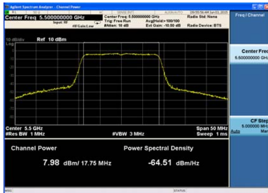
Ant : A1_802.11n_HT20 (1)
