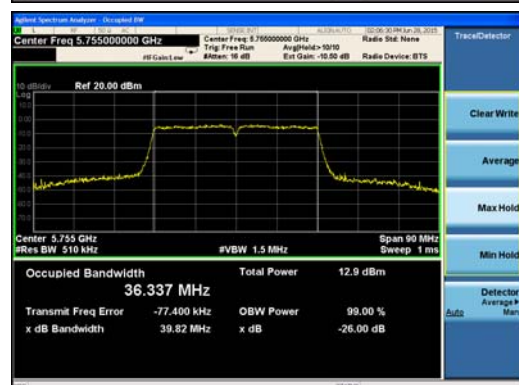
Ant : A3_802.11n_HT40 (1)
