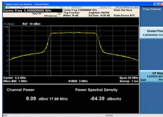
Ant : A2_802.11ac_VHT20 (1)
