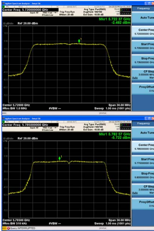
Ant : A2_802.11ac_VHT20 (2)
