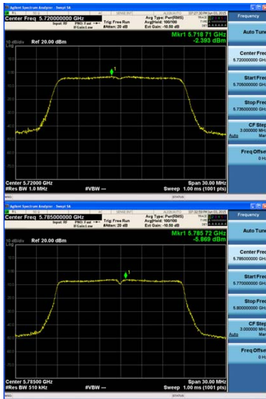
Ant : A3_802.11n_HT20 (2)
