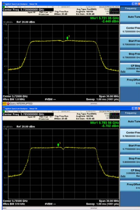
Ant : A2_802.11n_HT20 (2)
