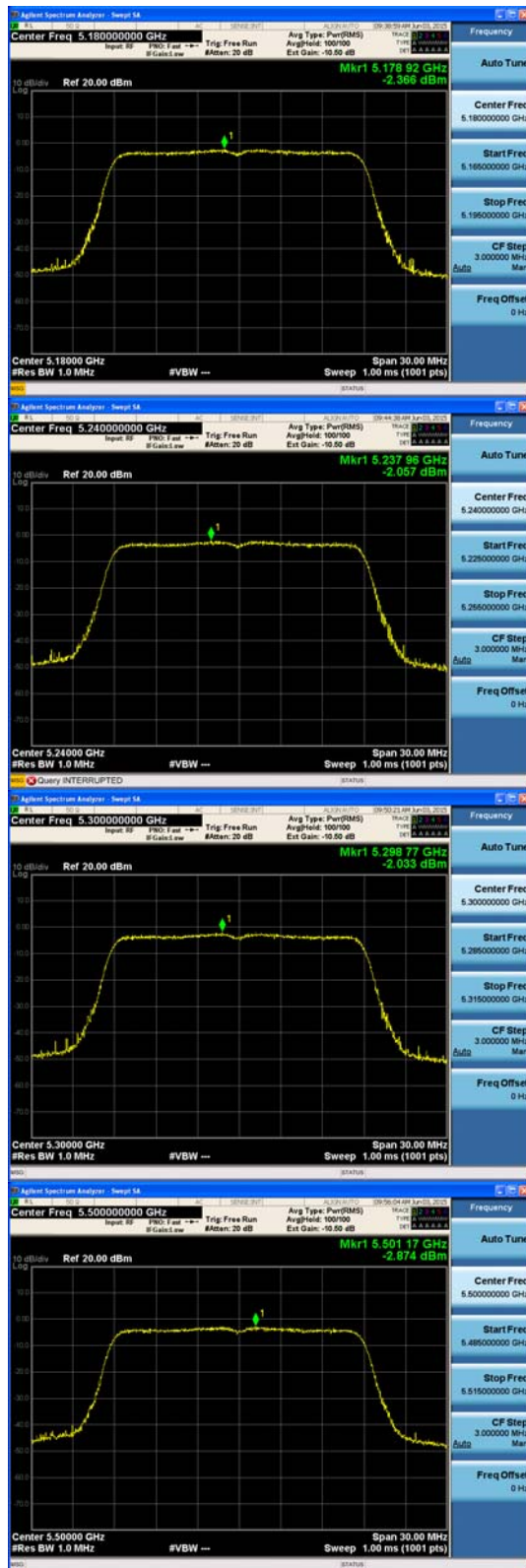
Ant : A1_802.11n_HT20 (1)
