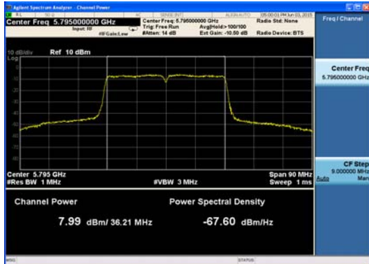
Ant : A2_802.11ac_HT40 (2)
