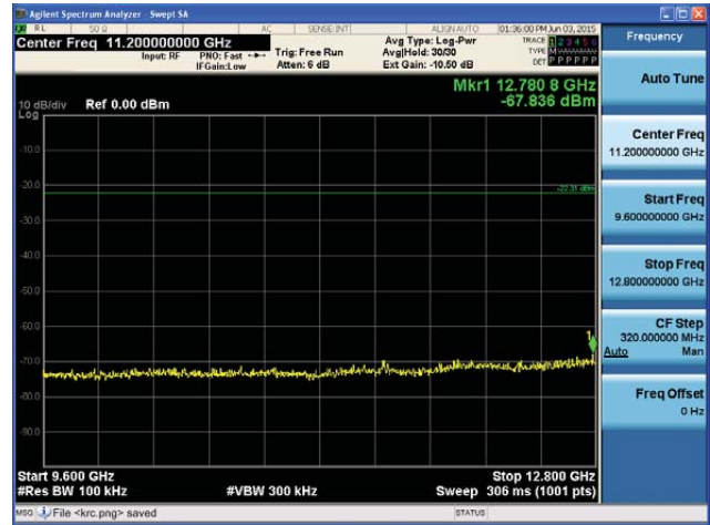
5785MHz 9.6GHz~12.8GHz
