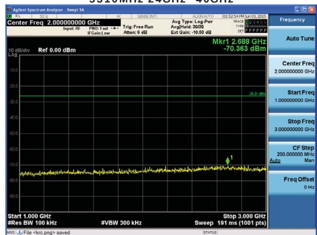
5510MHz 1GHz~3GHz
