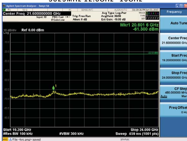
5825MHz 19.2GHz~24GHz
