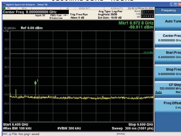
5230MHz 6.4GHz~9.6GHz
