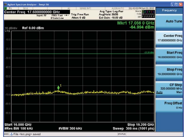
5190MHz 16GHz~19.2GHz
