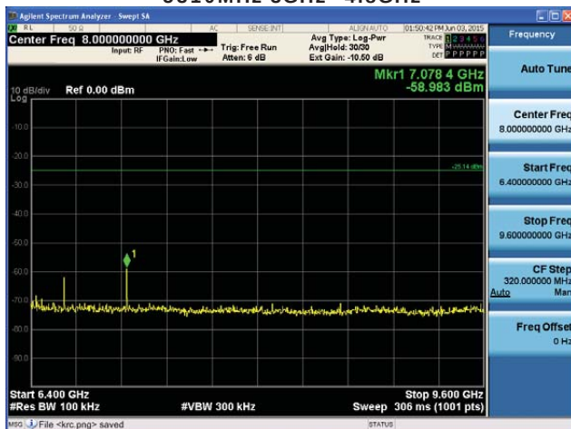
5310MHz 6.4GHz~9.6GHz
