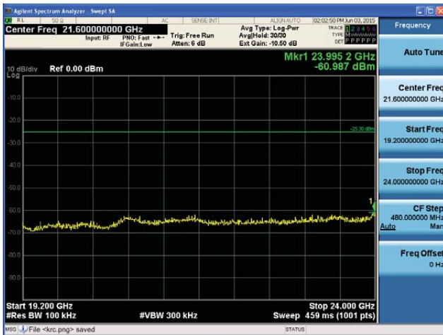
5755MHz 19.2GHz~24GHz
