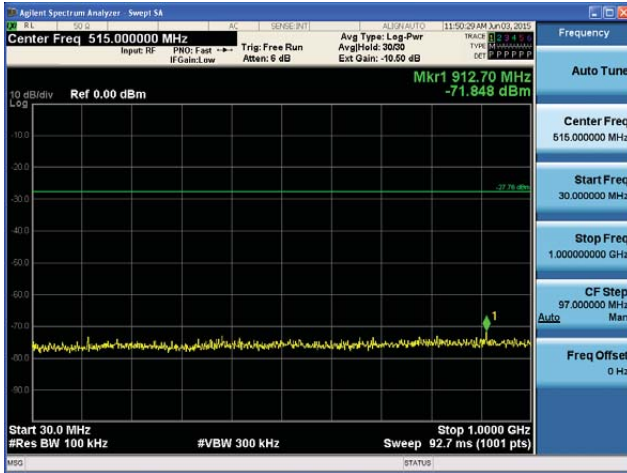
5210MHz 30MHz~1GHz
