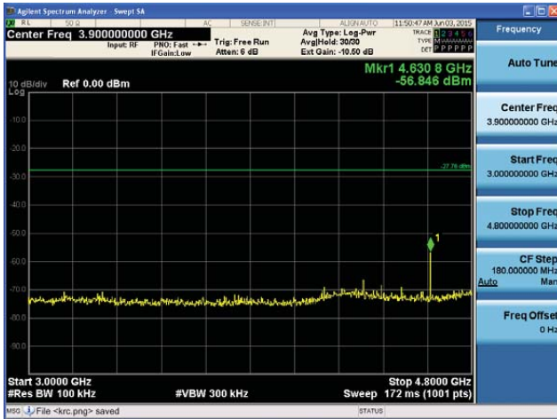
5210MHz 3GHz~4.8GHz
