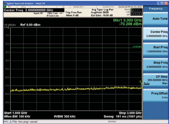
5795MHz 1GHz~3GHz
