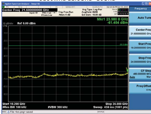
5180MHz 19.2GHz~24GHz
