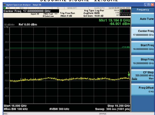
5290MHz 16GHz~19.2GHz
