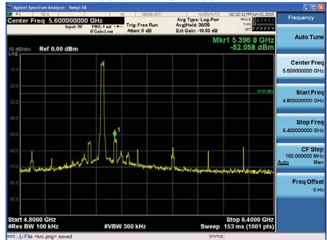
5320MHz 4.8GHz~6.4GHz
