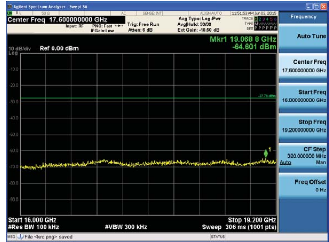
5210MHz 16GHz~19.2GHz
