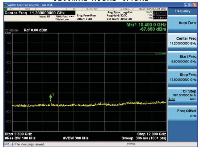
5200MHz 9.6GHz~12.8GHz
