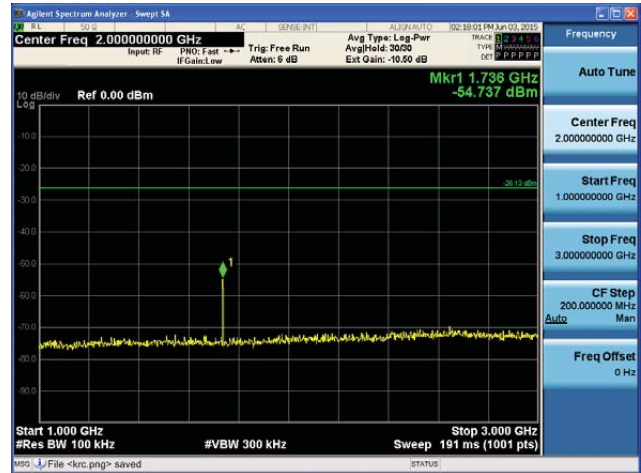
5180MHz 1GHz~3GHz
