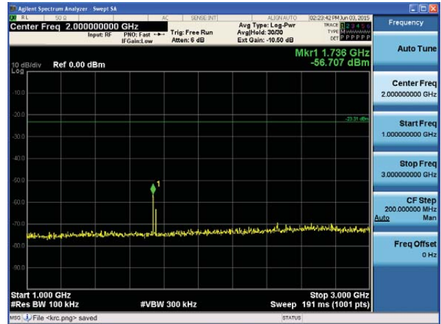
5240MHz 1GHz~3GHz
