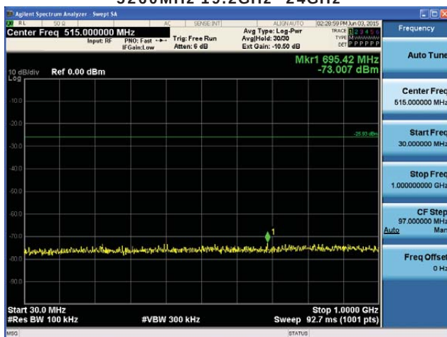
5300MHz 30MHz~1GHz
