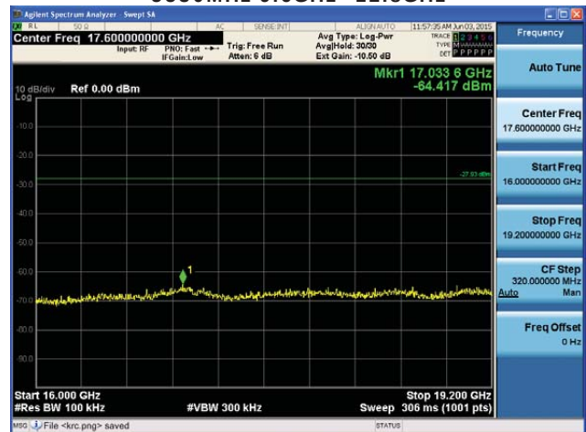
5530MHz 16GHz~19.2GHz
