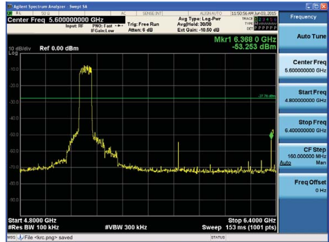
5210MHz 4.8GHz~6.4GHz
