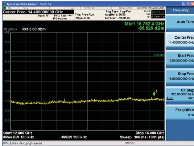
5320MHz 12.8GHz~16GHz
