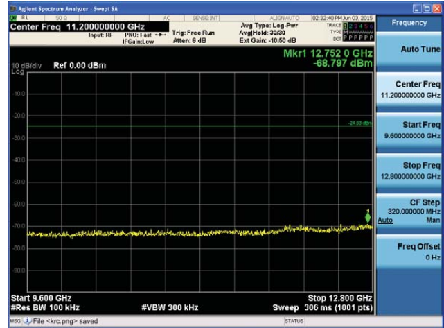
5320MHz 9.6GHz~12.8GHz
