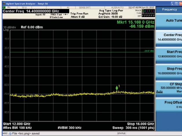
5720MHz 12.8GHz~16GHz
