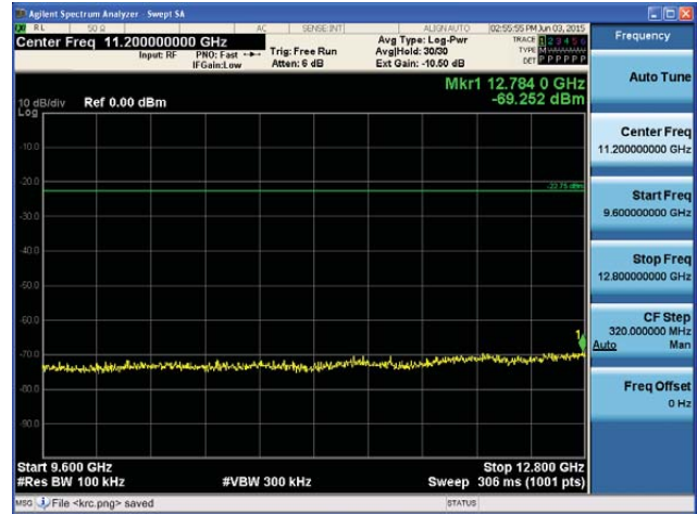
5825MHz 9.6GHz~12.8GHz
