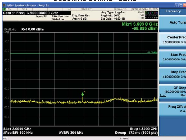
5825MHz 3GHz~4.8GHz
