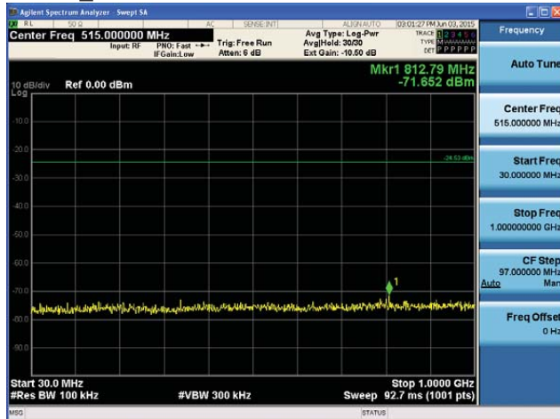
5180MHz 30MHz~1GHz
