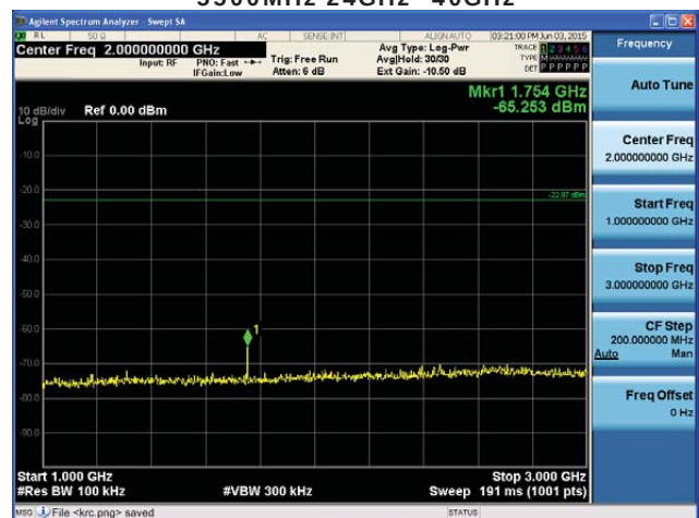
5600MHz 1GHz~3GHz
