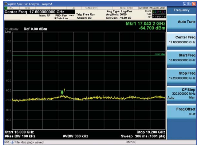
5720MHz 16GHz~19.2GHz
