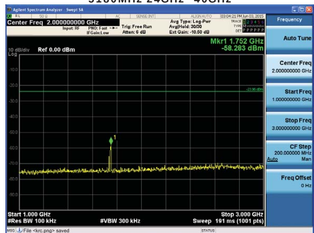
5200MHz 1GHz~3GHz
