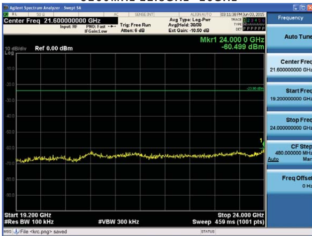
5260MHz 19.2GHz~24GHz
