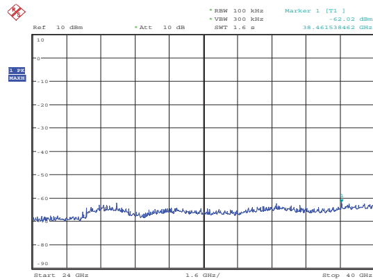
5600MHz 24GHz~40GHz
