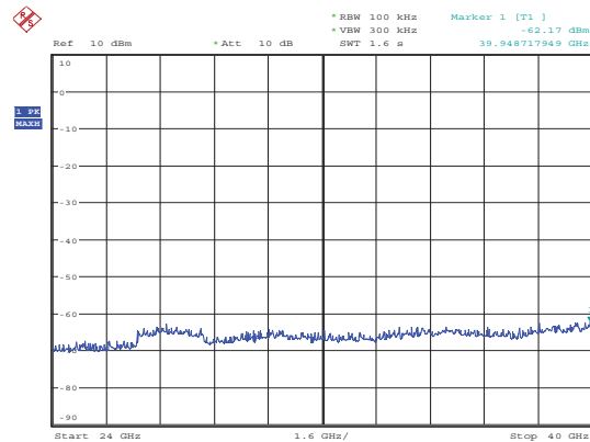
5755MHz 24GHz~40GHz
