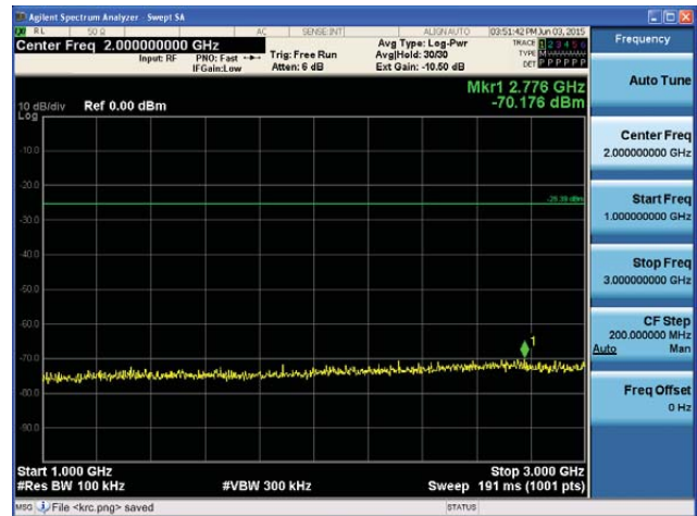
5710MHz 1GHz~3GHz
