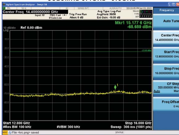
5825MHz 12.8GHz~16GHz
