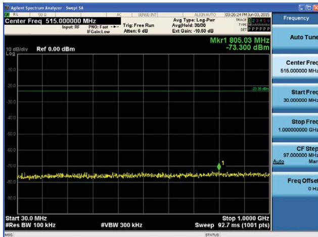
5745MHz 30MHz~1GHz
