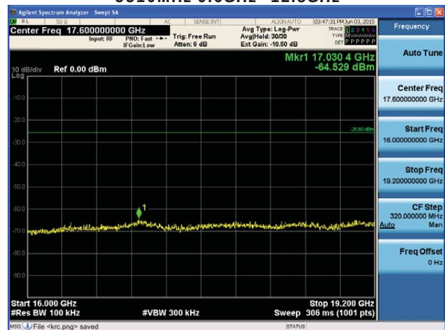
5510MHz 16GHz~19.2GHz
