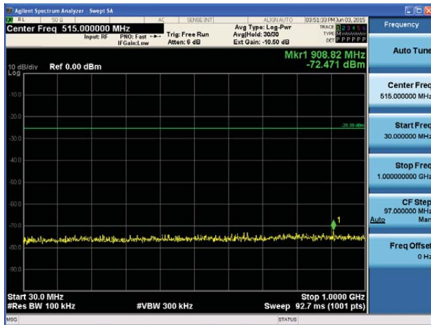
5710MHz 30MHz~1GHz
