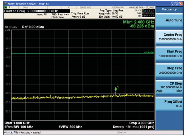
5270MHz 1GHz~3GHz
