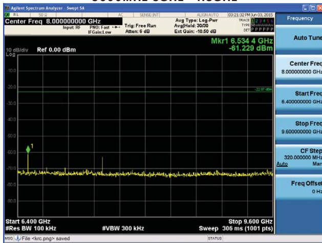
5600MHz 6.4GHz~9.6GHz
