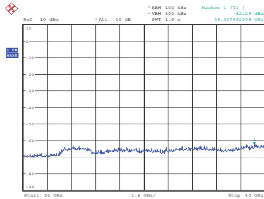
5510MHz 24GHz~40GHz
