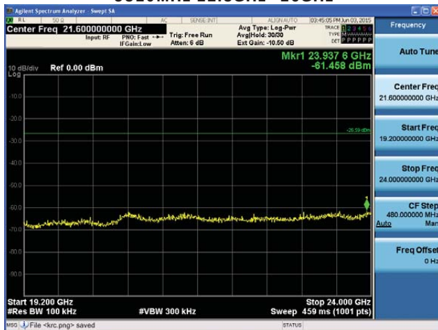
5310MHz 19.2GHz~24GHz
