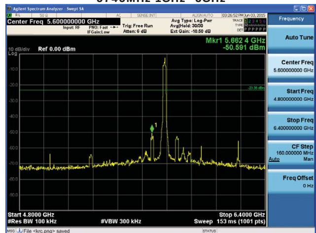
5745MHz 4.8GHz~6.4GHz
