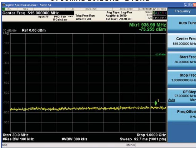
5825MHz 30MHz~1GHz
