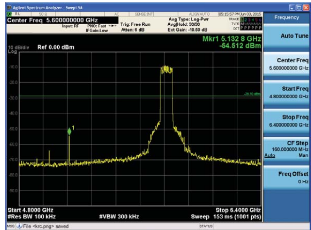
5775MHz 4.8GHz~6.4GHz
