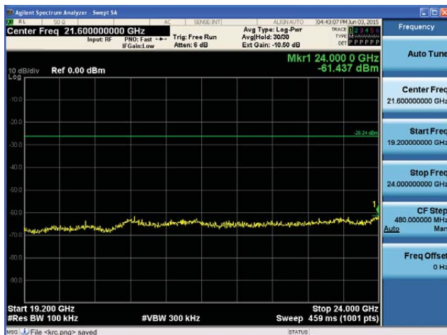
5230MHz 19.2GHz~24GHz
