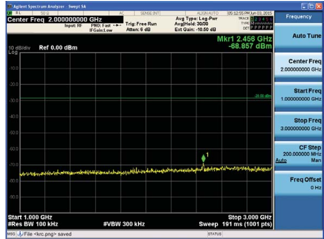
5690MHz 1GHz~3GHz
