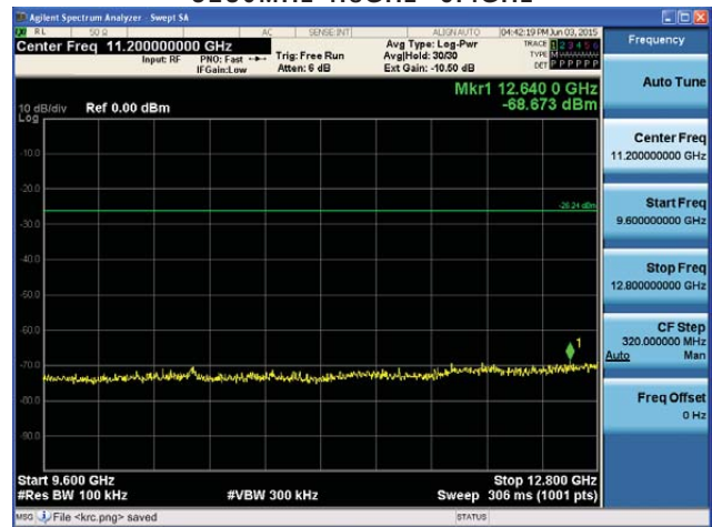
5230MHz 9.6GHz~12.8GHz
