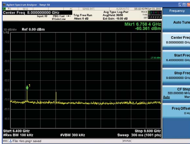
5530MHz 6.4GHz~9.6GHz
