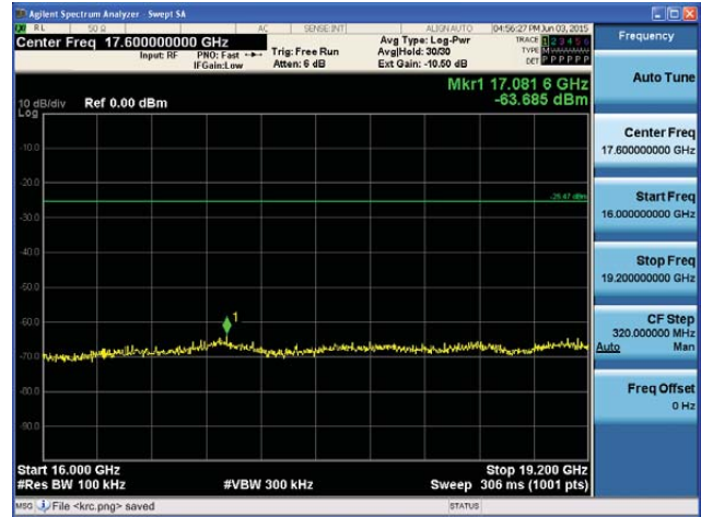
5710MHz 16GHz~19.2GHz
