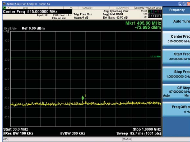
5530MHz 30MHz~1GHz
