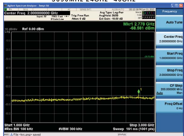
5775MHz 1GHz~3GHz
