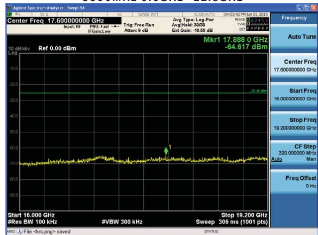
5590MHz 16GHz~19.2GHz
