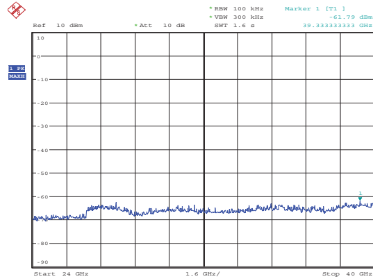
5755MHz 24GHz~40GHz
