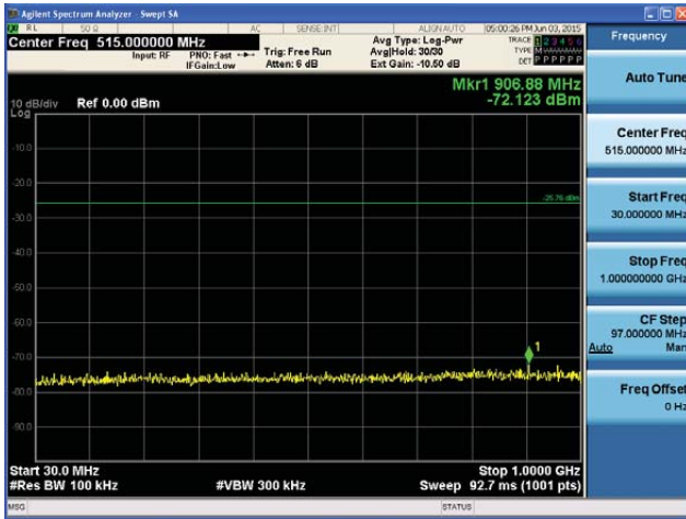
5795MHz 30MHz~1GHz
