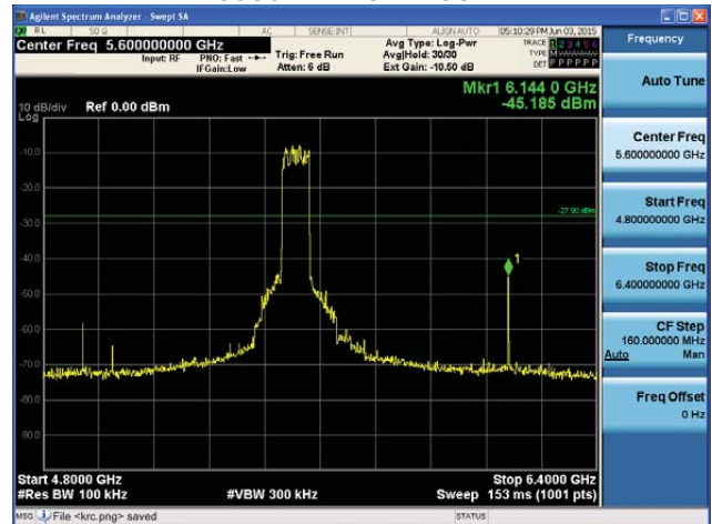
5530MHz 4.8GHz~6.4GHz
