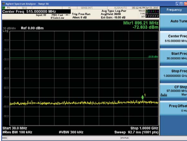
5690MHz 30MHz~1GHz
