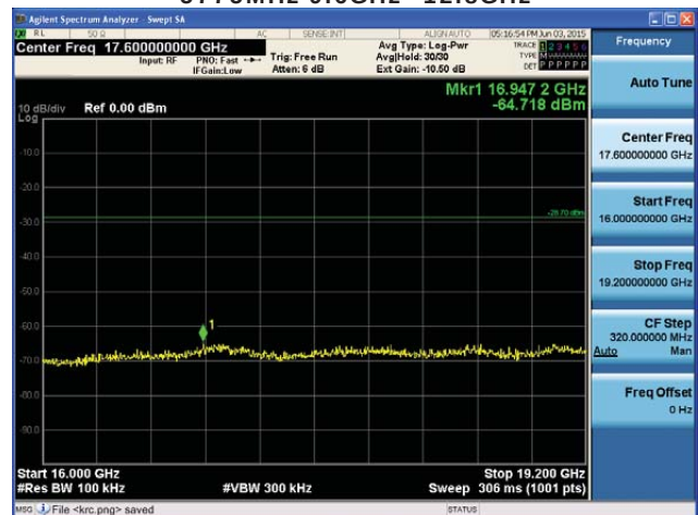
5775MHz 16GHz~19.2GHz
