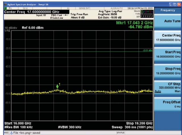
5260MHz 16GHz~19.2GHz
