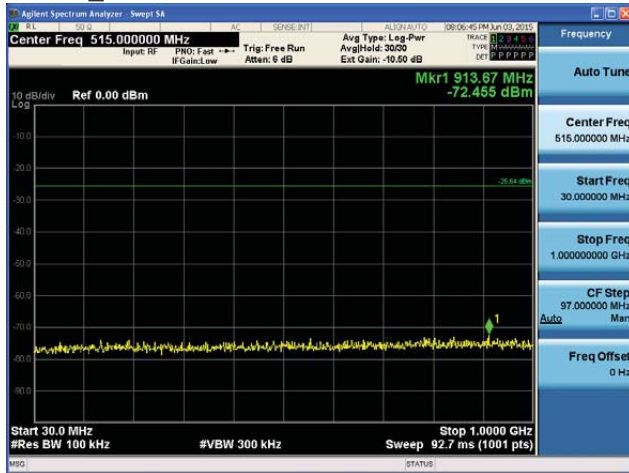
5180MHz 30MHz~1GHz
