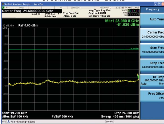
5710MHz 19.2GHz~24GHz
