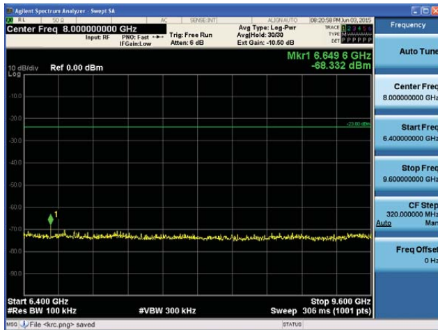
5320MHz 6.4GHz~9.6GHz
