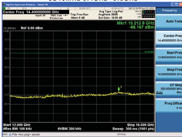
5240MHz 12.8GHz~16GHz
