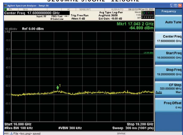
5200MHz 16GHz~19.2GHz
