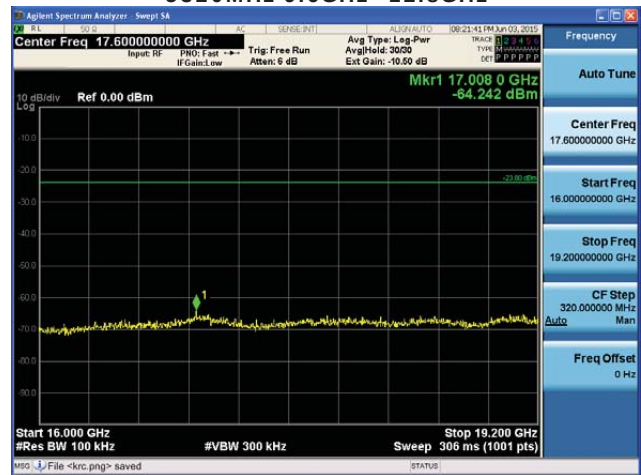
5320MHz 16GHz~19.2GHz
