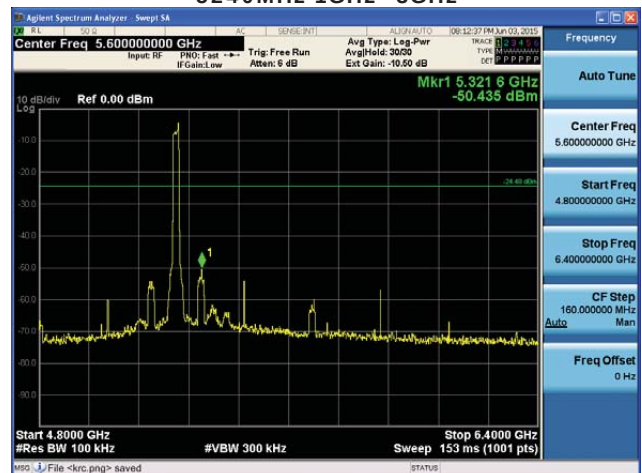
5240MHz 4.8GHz~6.4GHz
