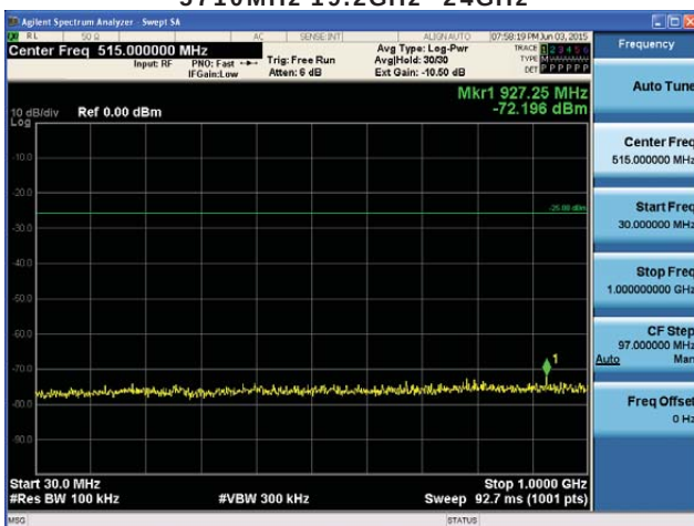
5755MHz 30MHz~1GHz
