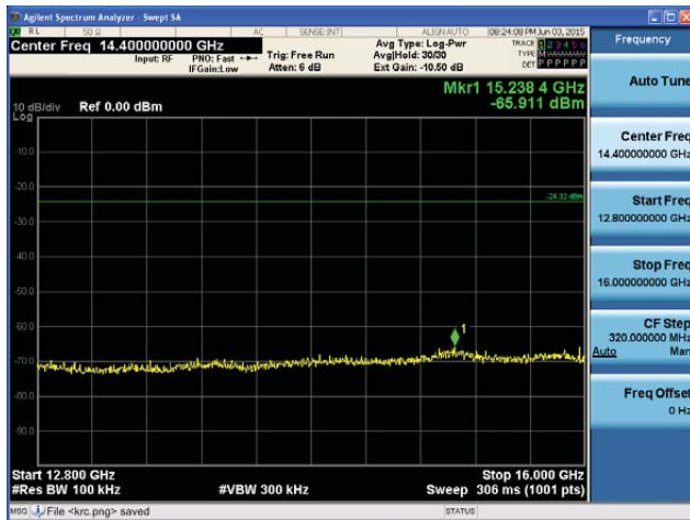
5500MHz 12.8GHz~16GHz
