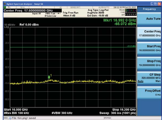
5745MHz 16GHz~19.2GHz
