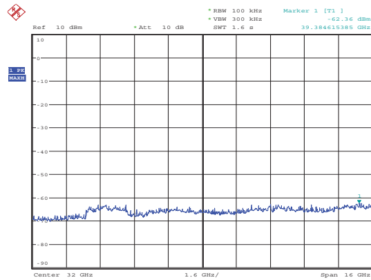
5785MHz 24GHz~40GHz
