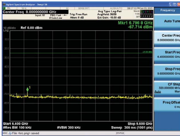
5825MHz 6.4GHz~9.6GHz
