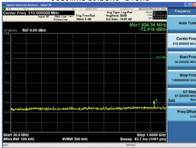
5590MHz 30MHz~1GHz
