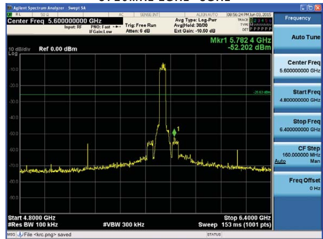
5710MHz 4.8GHz~6.4GHz
