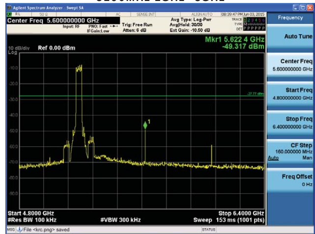
5190MHz 4.8GHz~6.4GHz
