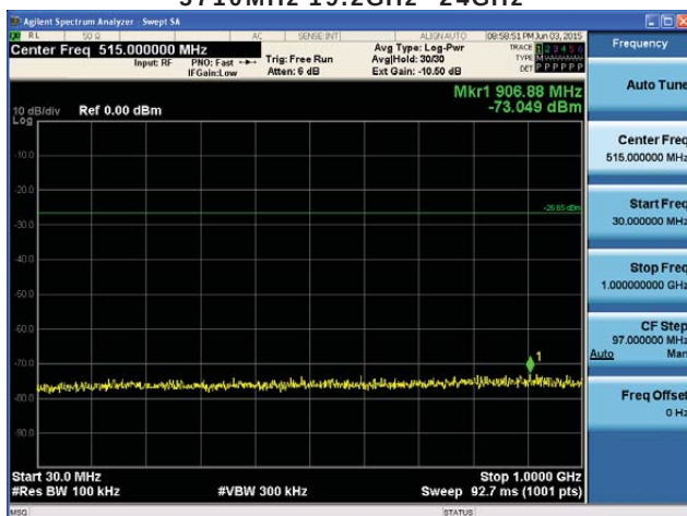
5755MHz 30MHz~1GHz
