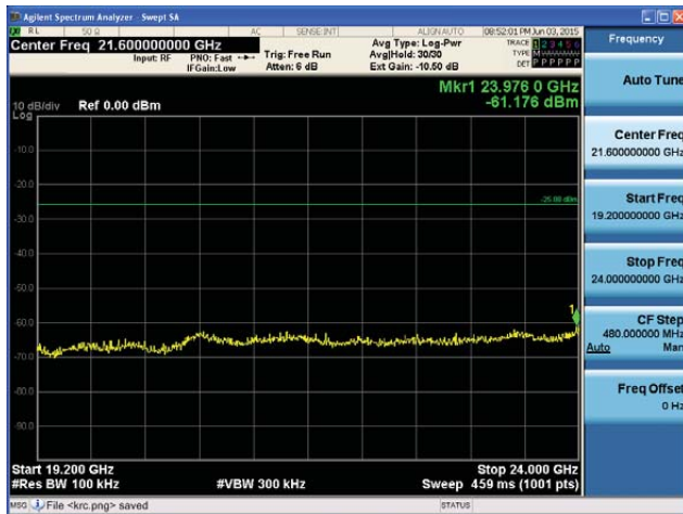
5510MHz 19.2GHz~24GHz
