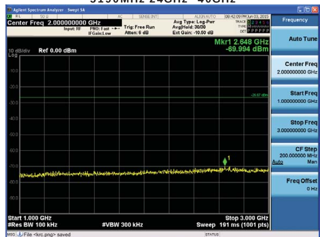
5230MHz 1GHz~3GHz
