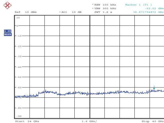
5510MHz 24GHz~40GHz
