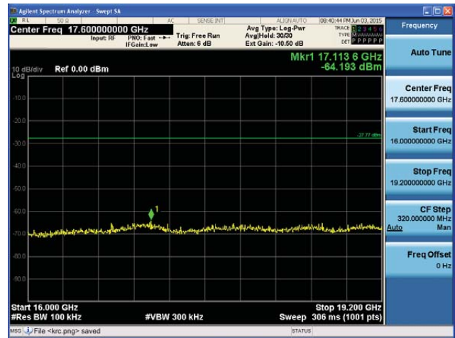
5190MHz 16GHz~19.2GHz
