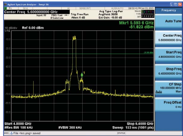
5510MHz 4.8GHz~6.4GHz
