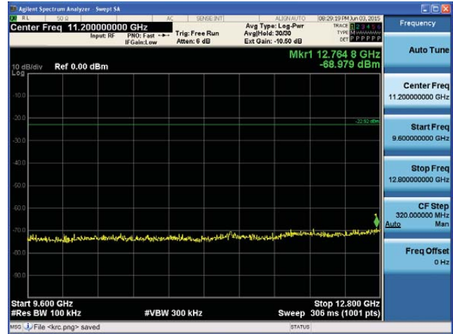
5720MHz 9.6GHz~12.8GHz
