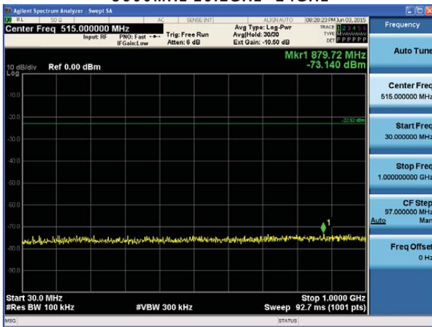
5720MHz 30MHz~1GHz
