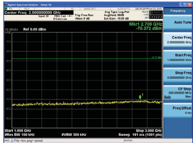
5190MHz 1GHz~3GHz
