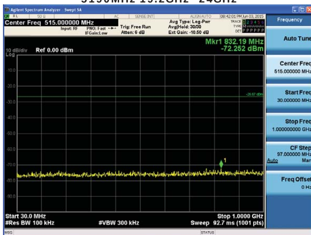
5230MHz 30MHz~1GHz
