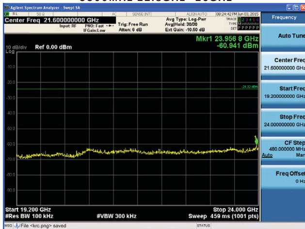
5500MHz 19.2GHz~24GHz
