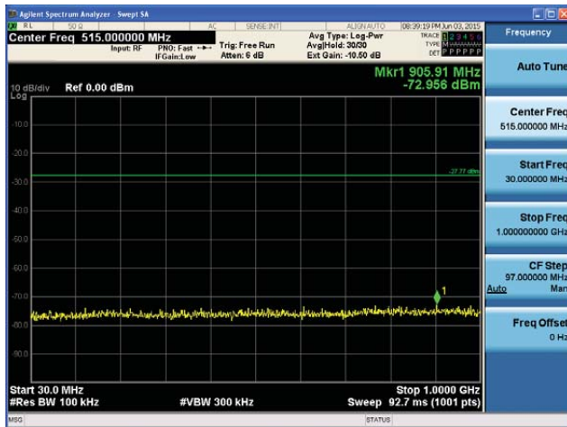
5190MHz 30MHz~1GHz
