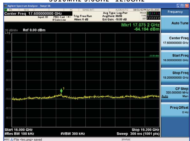
5510MHz 16GHz~19.2GHz
