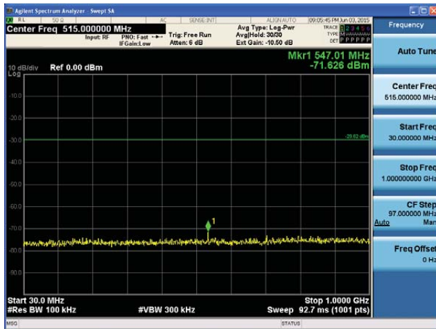
5210MHz 30MHz~1GHz
