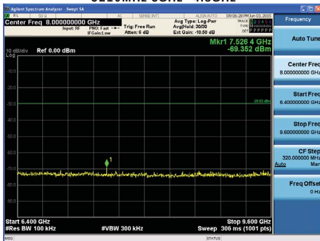
5210MHz 6.4GHz~9.6GHz
