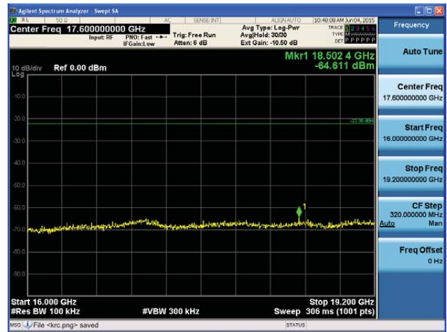
5180MHz 16GHz~19.2GHz
