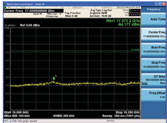
5690MHz 16GHz~19.2GHz
