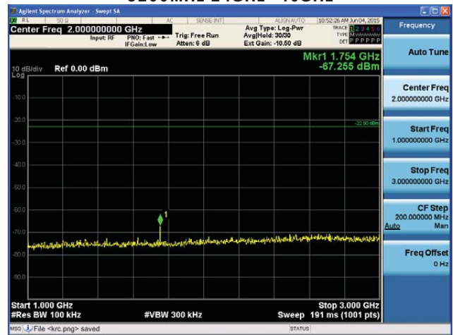
5240MHz 1GHz~3GHz
