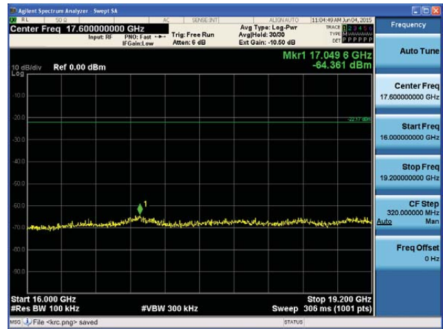
5500MHz 16GHz~19.2GHz
