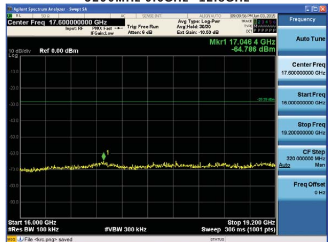
5290MHz 16GHz~19.2GHz
