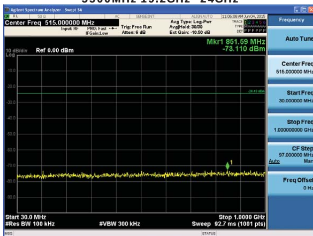
5600MHz 30MHz~1GHz
