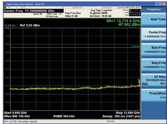
5320MHz 9.6GHz~12.8GHz
