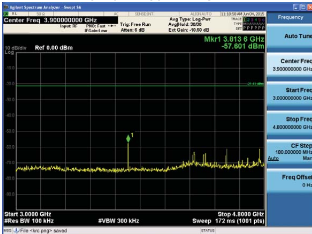
5720MHz 3GHz~4.8GHz
