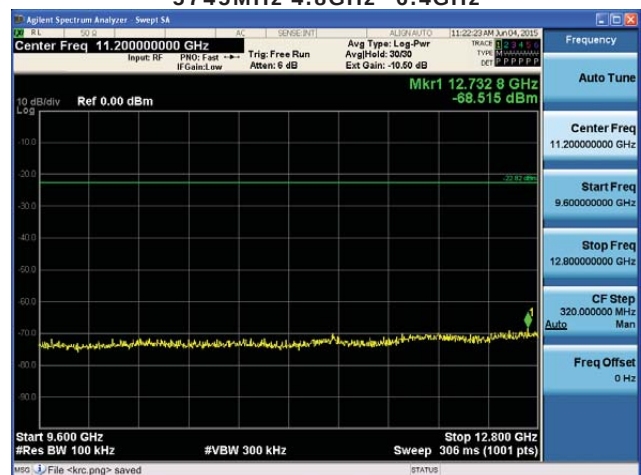
5745MHz 9.6GHz~12.8GHz
