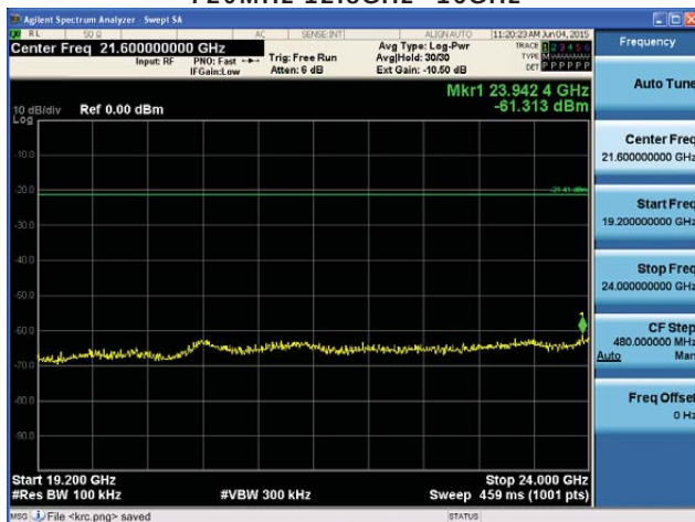
5720MHz 19.2GHz~24GHz
