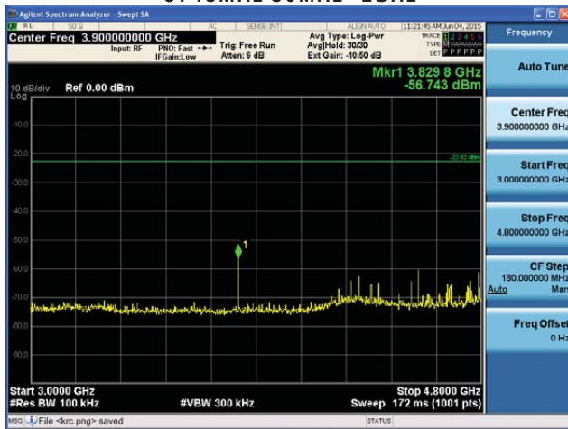
5745MHz 3GHz~4.8GHz
