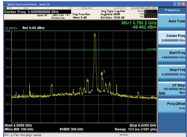
5720MHz 4.8GHz~6.4GHz
