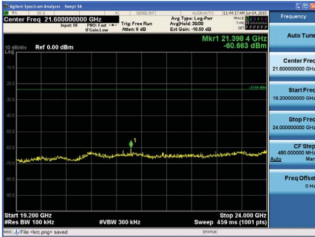
5300MHz 19.2GHz~24GHz
