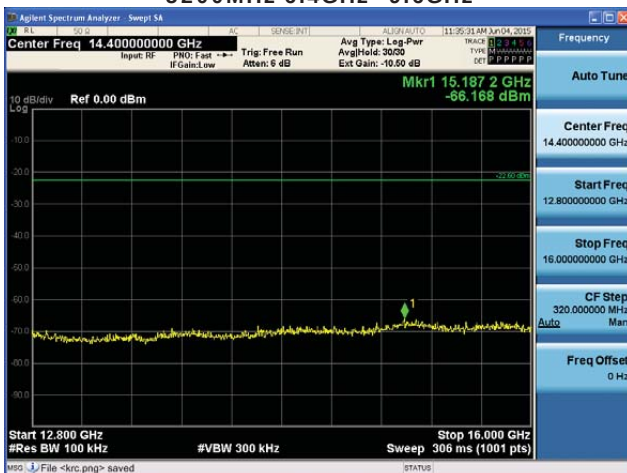
5200MHz 12.8GHz~16GHz
