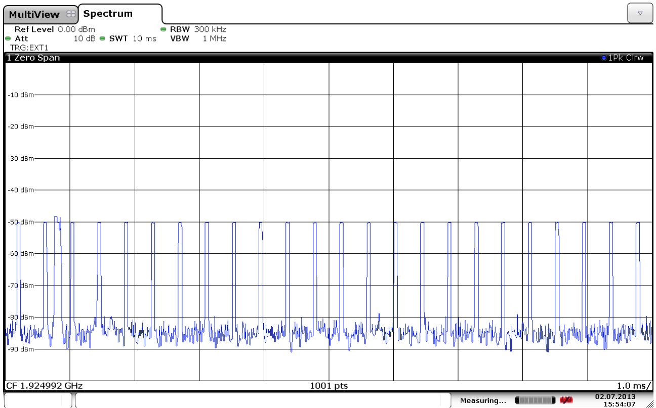
50 µs Pulses
