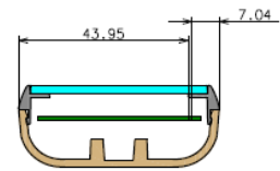
Sec. B-B (Pattern antenna)
