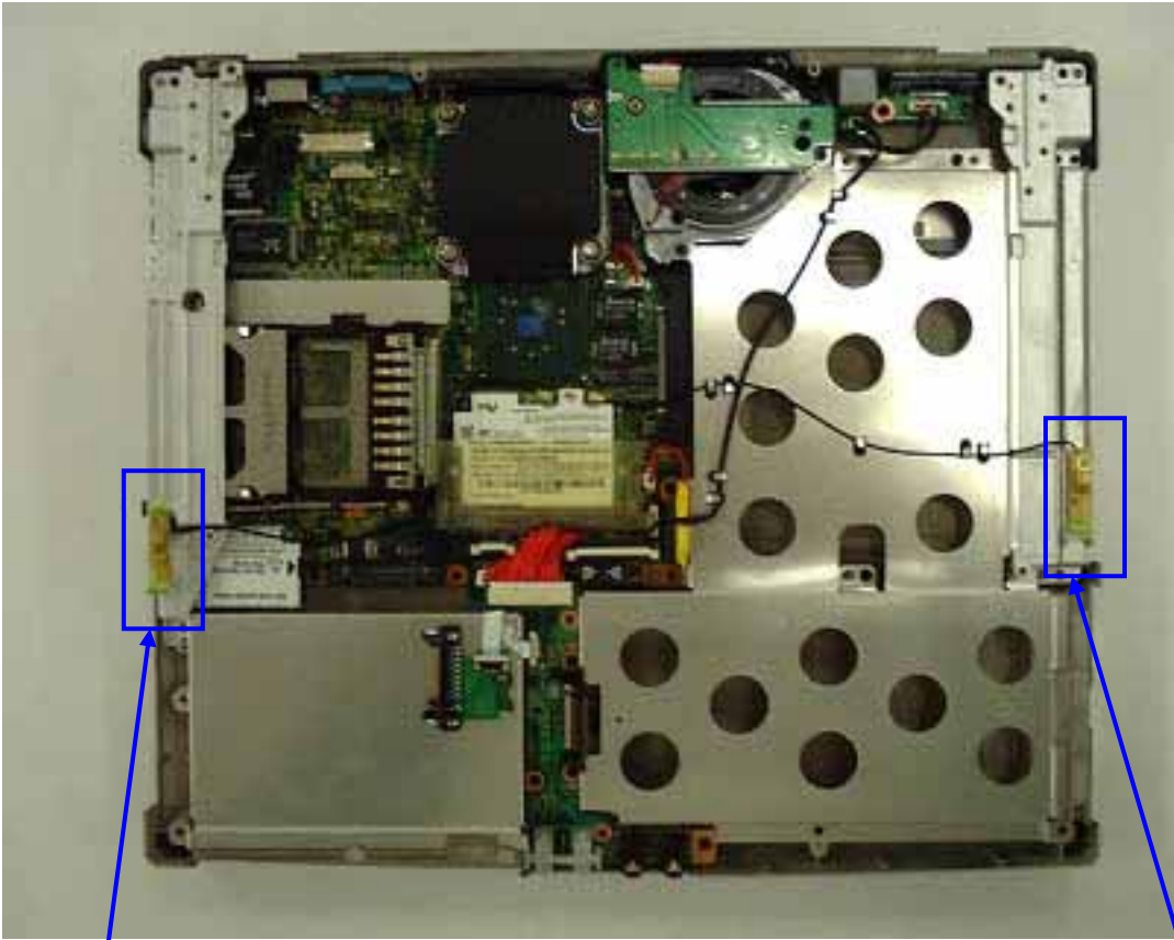
Left TX/RX Antenna
