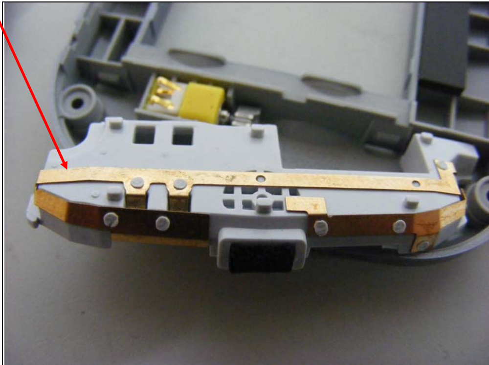
GSM Antenna
